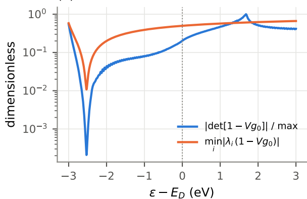
(d) resonance criterion
