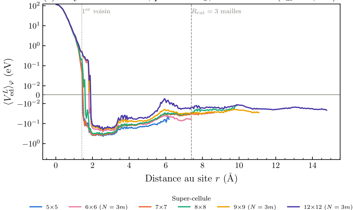
(c) Moyenne azimutale, plan z = z_C , cœurs exclus ( r_{at} < 0,5 Å)
