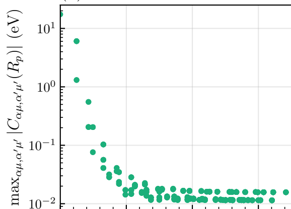
(b) C : constantes de force
