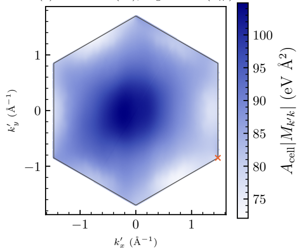
(d) conduction ( \pi^* ), align  exact ( F_W )
