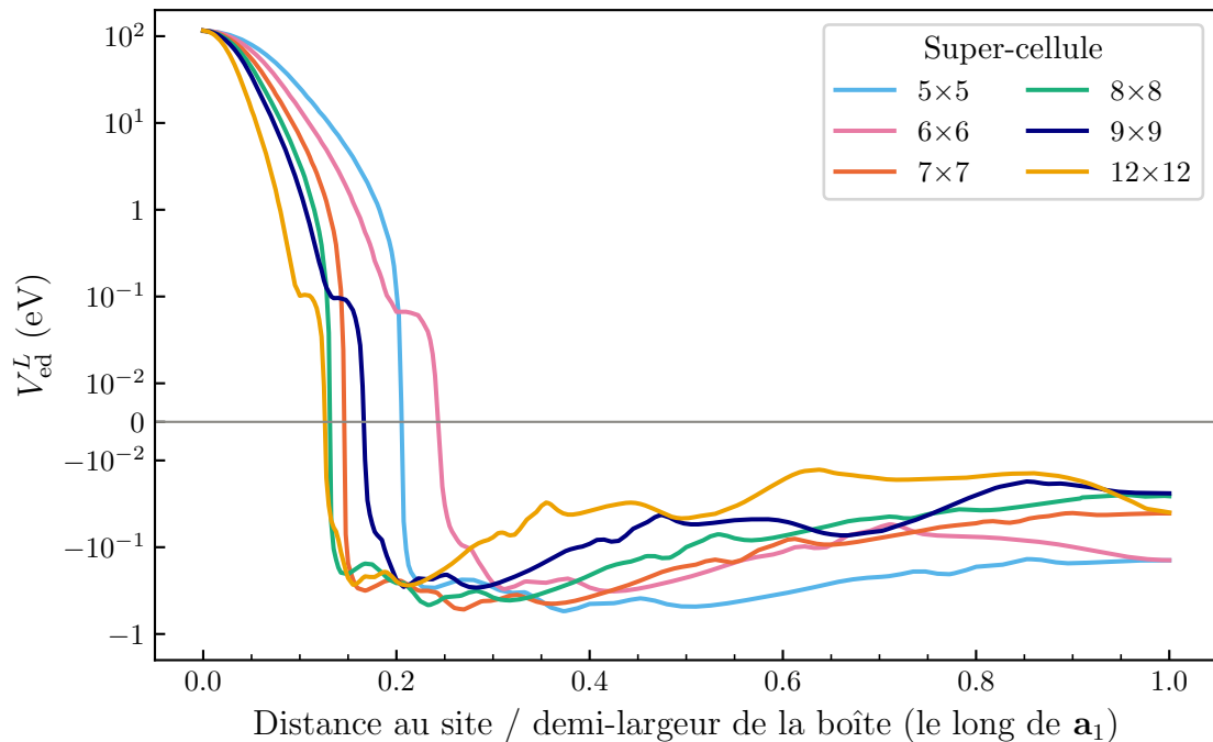
Potentiel de défaut local, du site de la lacune à la frontière
