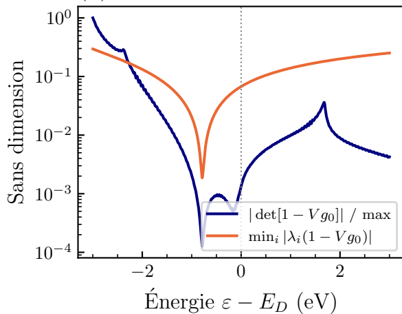
(d) Critère de résonance
