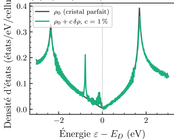
(d) Critère de résonance
