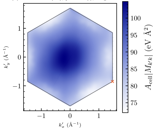
(d) conduction ( \pi^* ), plateau (i), Wigner-Seitz
