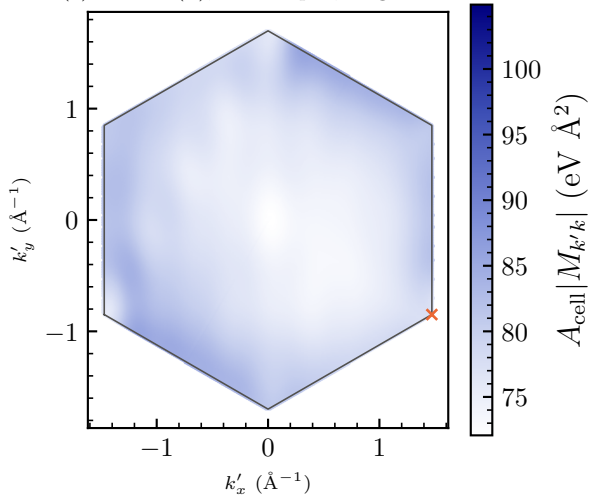
(a) valence ( \pi ), M2 tel quel, Wigner-Seitz
