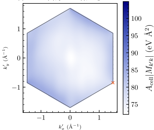
(c) valence ( \pi ), plateau (i), Wigner-Seitz
