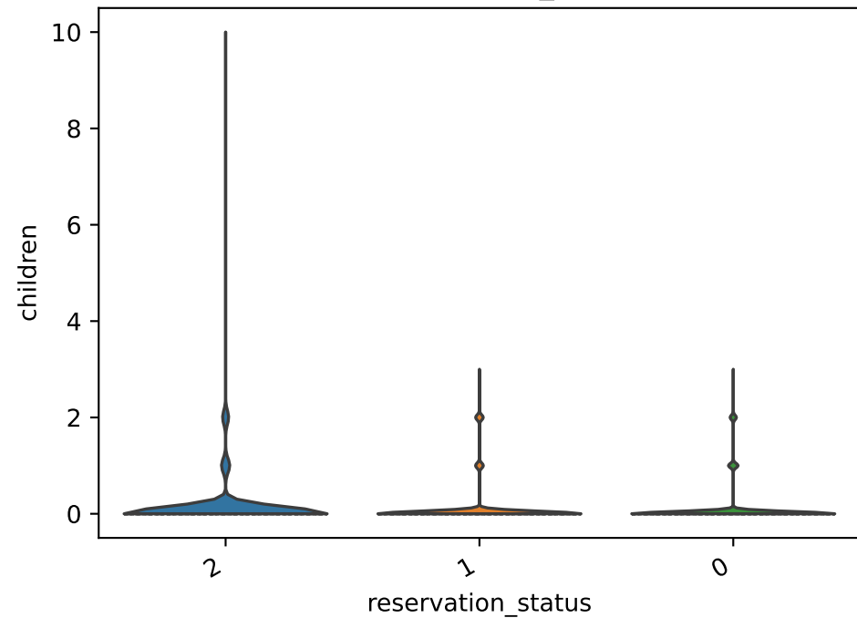
children par reservation_status (violins)
