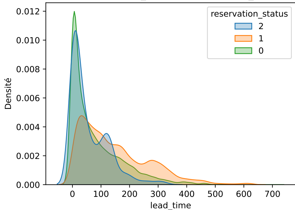
Densités de lead_time par reservation_status
