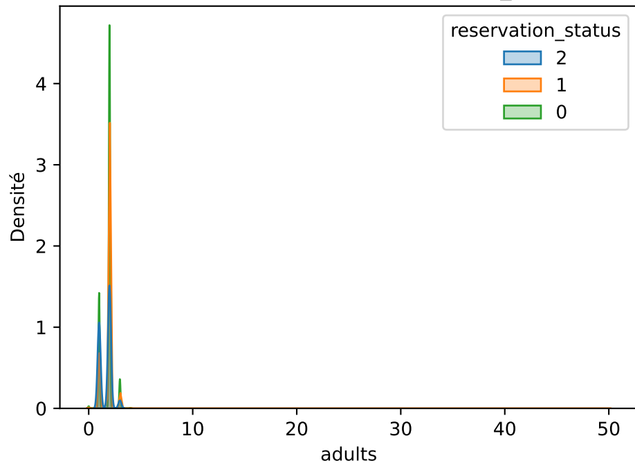
Densités de adults par reservation_status
