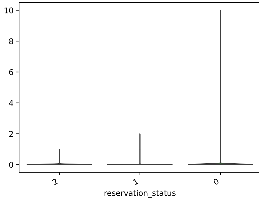
babies par reservation_status (violins)
