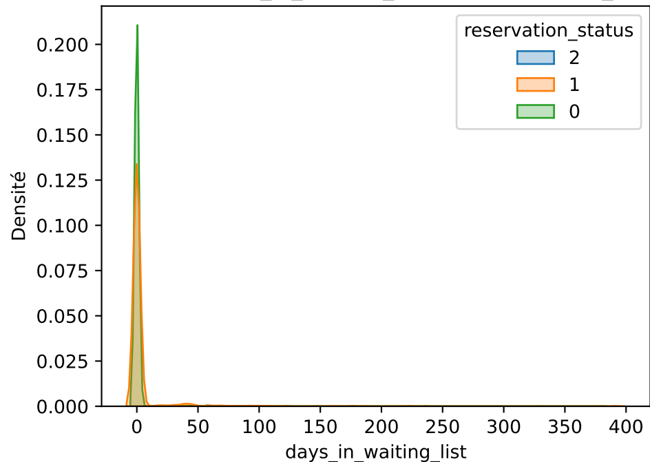
Densités de days_in_waiting_list par reservation_status
