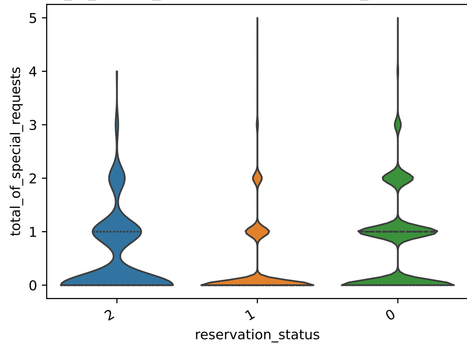
total_of_special_requests par reservation_status (violins) Densités de total_of_special_requests par reservation_status
