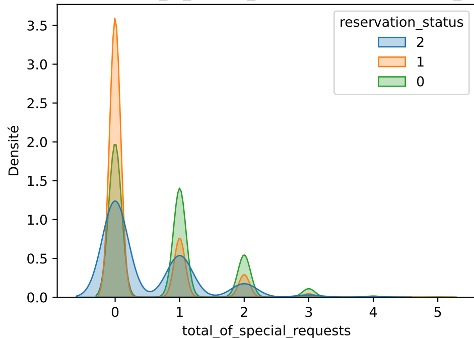
total_of_special_requests par reservation_status (violins) Densités de total_of_special_requests par reservation_status
