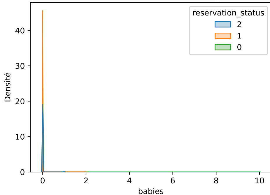
Densités de babies par reservation_status
