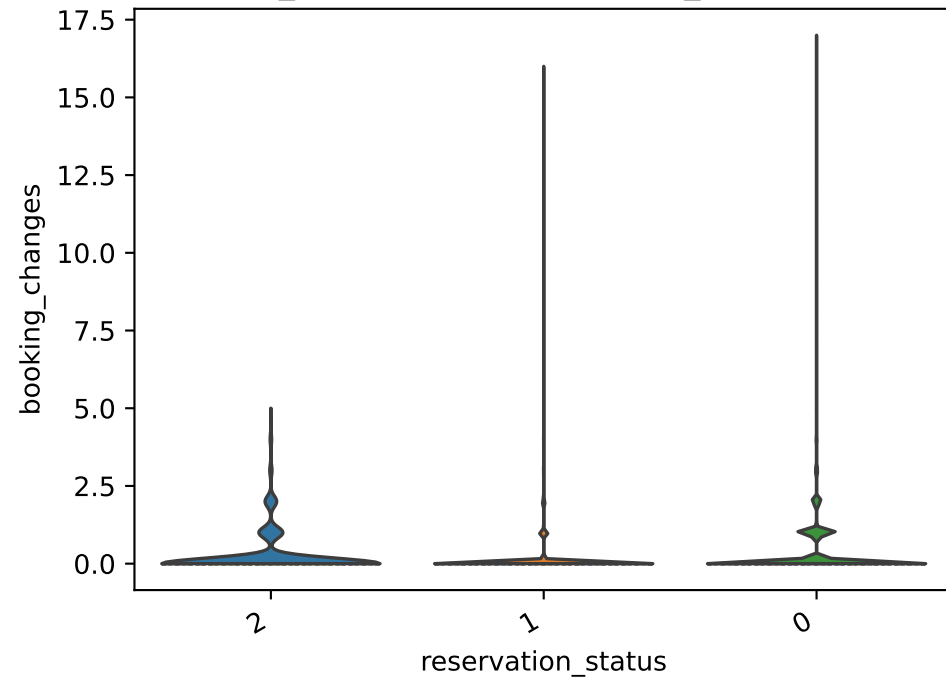
booking_changes par reservation_status (violins)
