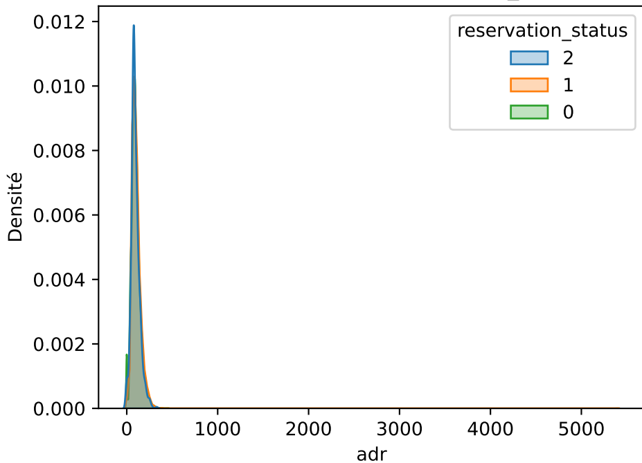
Densités de adr par reservation_status
