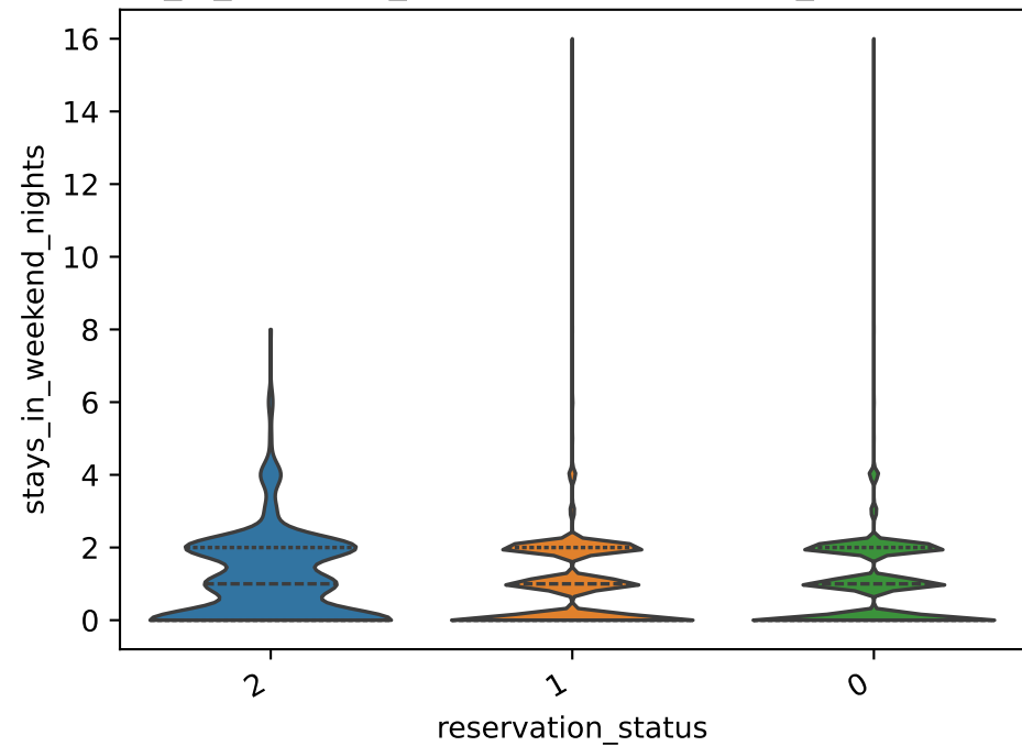
stays_in_weekend_nights par reservation_status (violins) Densités de stays_in_weekend_nights par reservation_status
