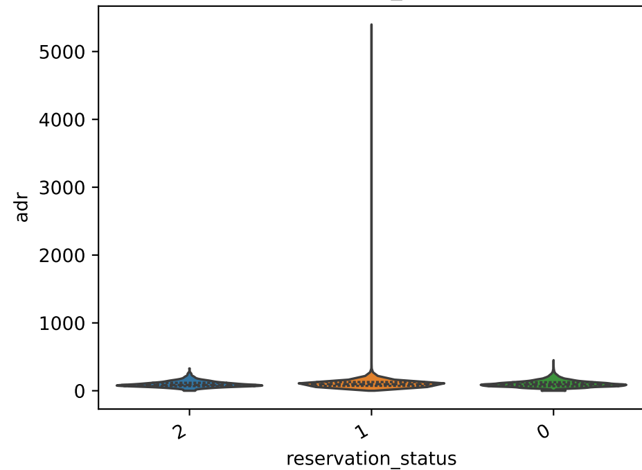
adr par reservation_status (violins)
