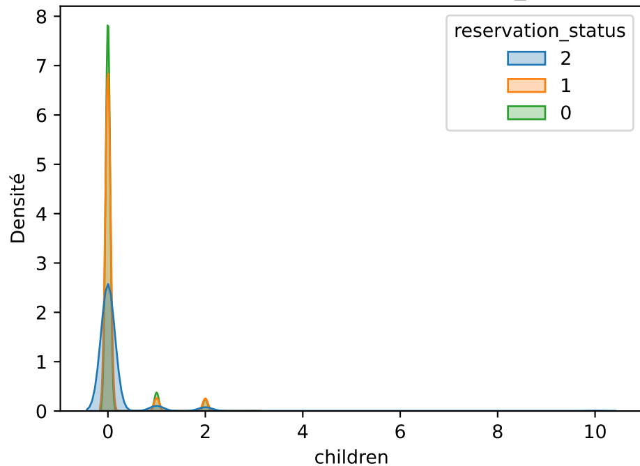
Densités de children par reservation_status
