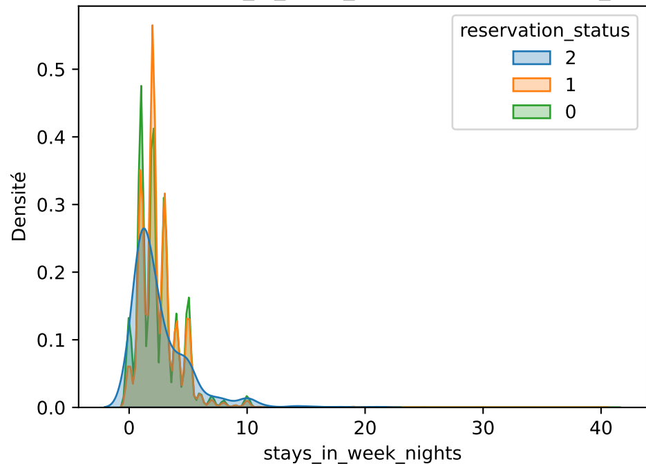
Densités de stays_in_week_nights par reservation_status
