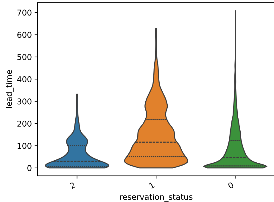
lead_time par reservation_status (violins)
