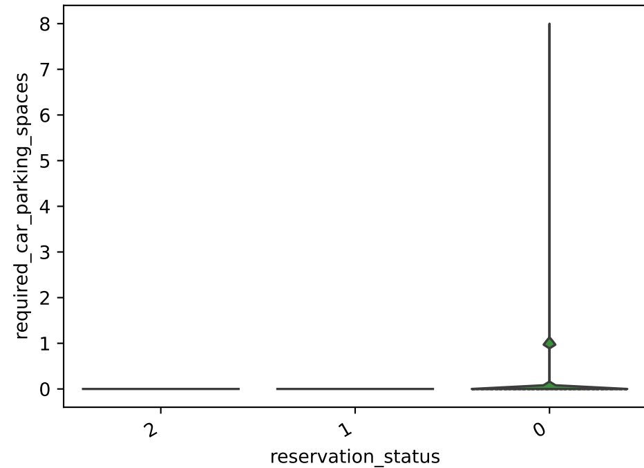
required_car_parking_spaces par reservation_status (violin) Densités de required_car_parking_spaces par reservation_status
