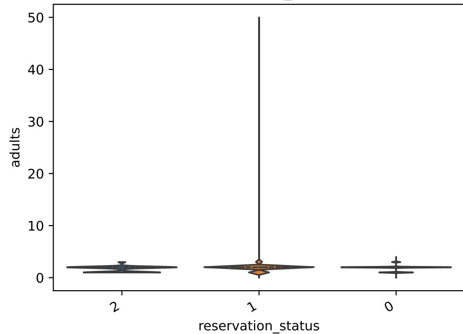
adults par reservation_status (violins)
