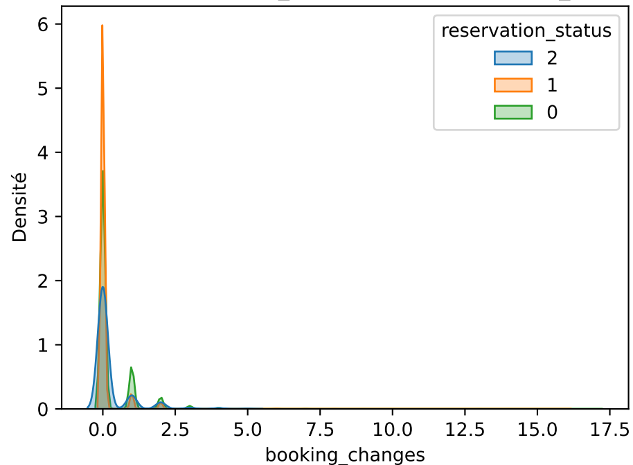
Densités de booking_changes par reservation_status
