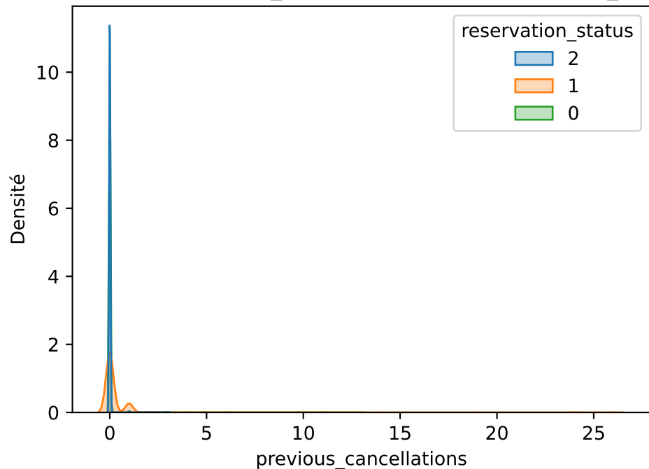
Densités de previous_cancellations par reservation_status
