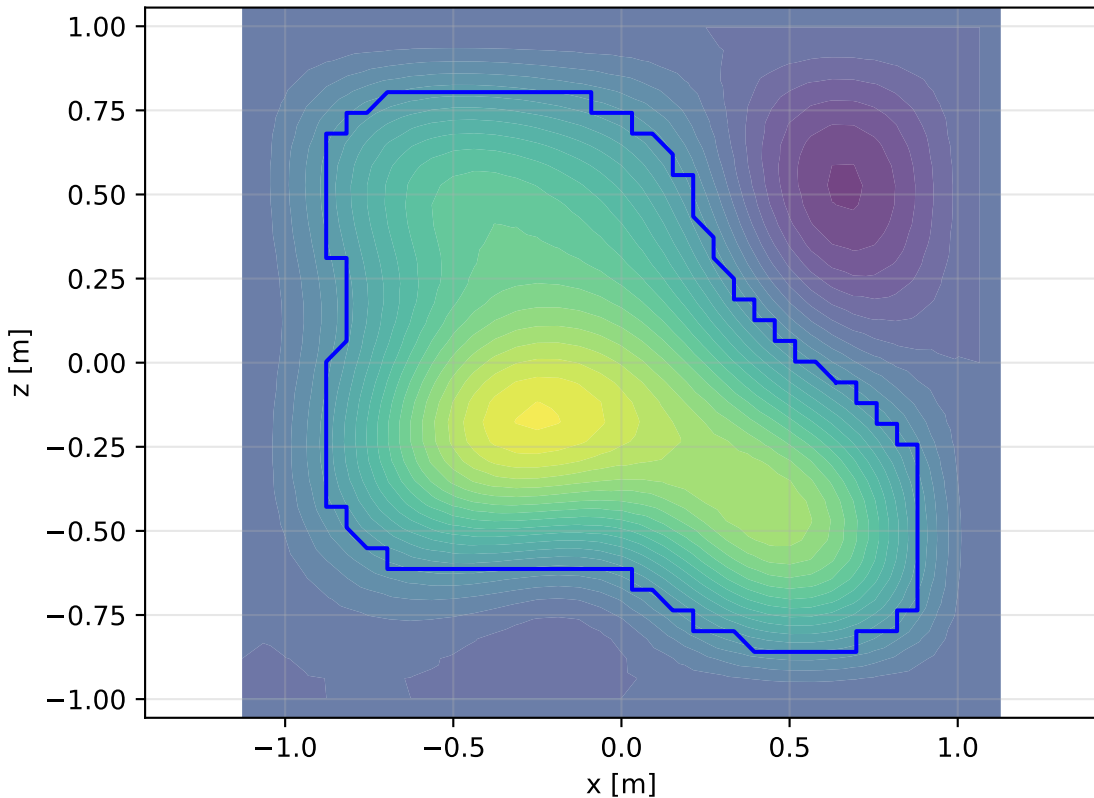
Face 3: xz-plane - Contour 3
