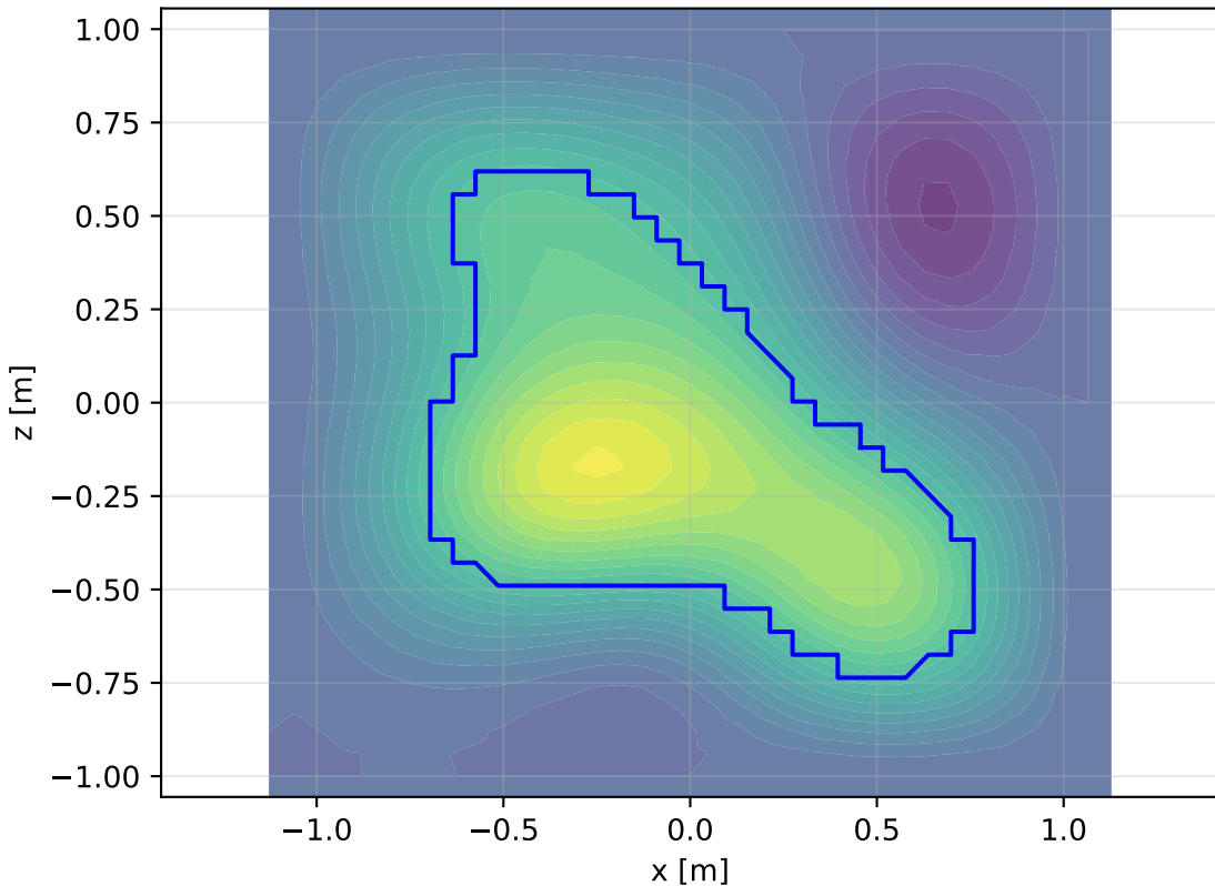
Face 3: xz-plane - Contour 5
