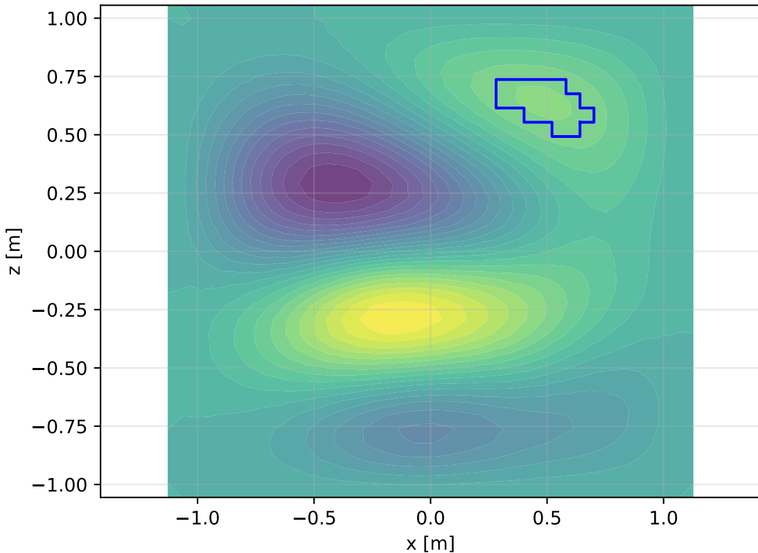
Face 4: xz-plane - Contour 20
