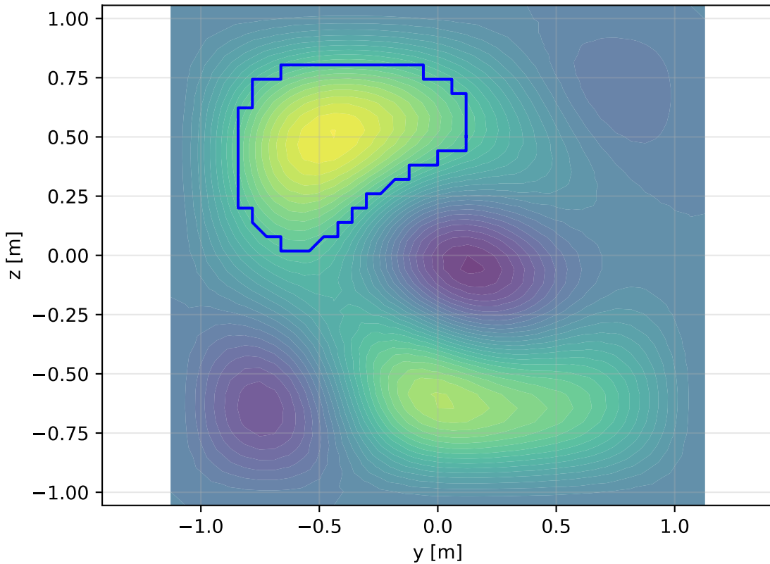
Face 5: yz-plane - Contour 12
