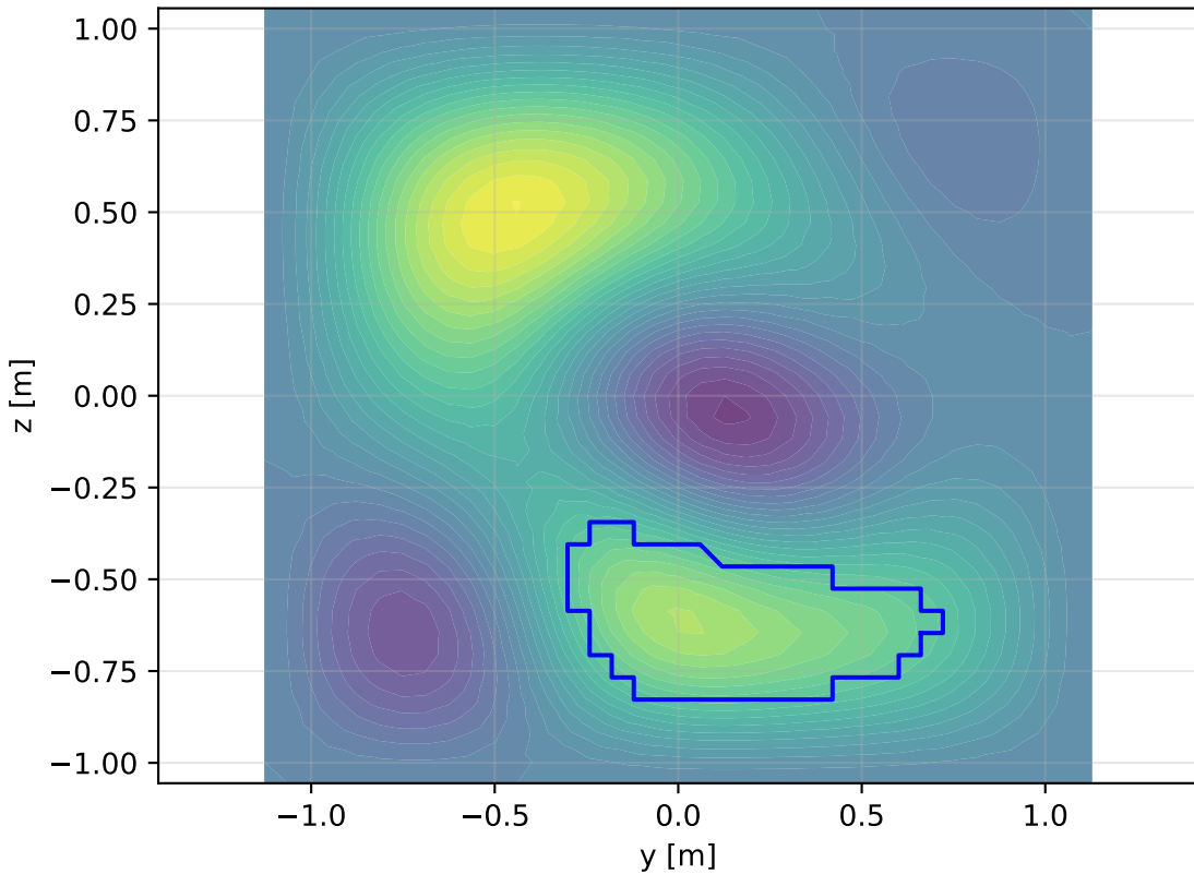
Face 5: yz-plane - Contour 13
