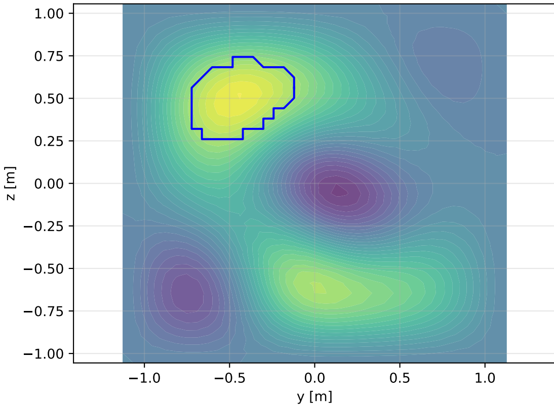
Face 5: yz-plane - Contour 16
