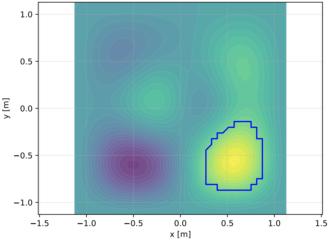
Face 1: xy-plane - Contour 19
