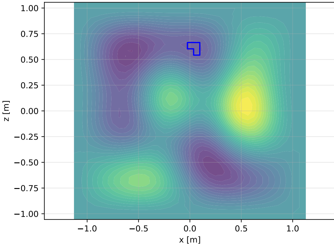
Face 3: xz-plane - Contour 1
