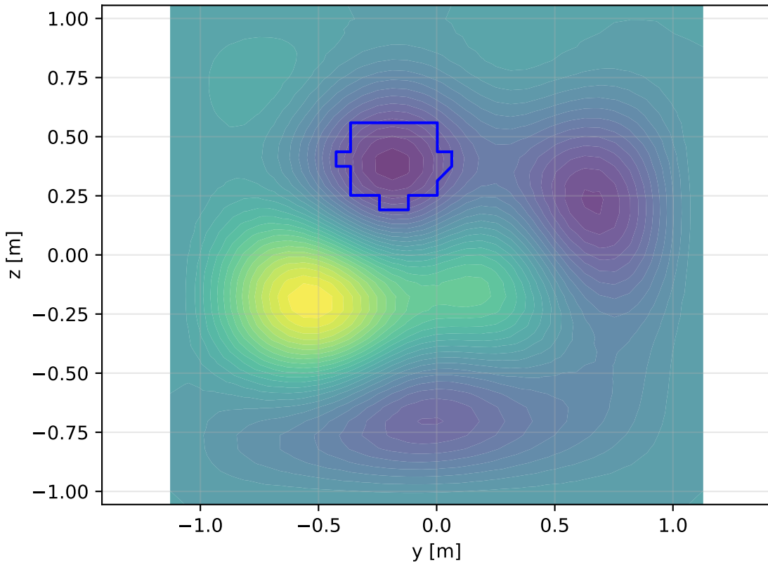
Face 5: yz-plane - Contour 2
