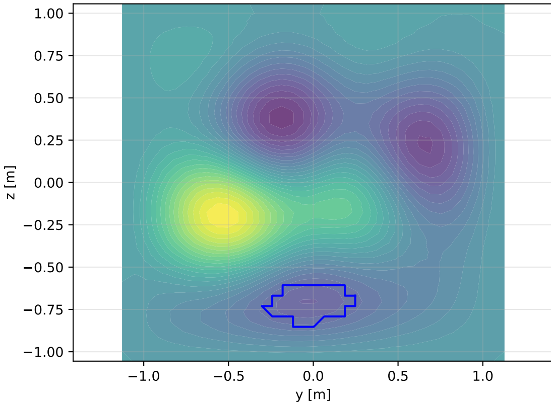
Face 5: yz-plane - Contour 5
