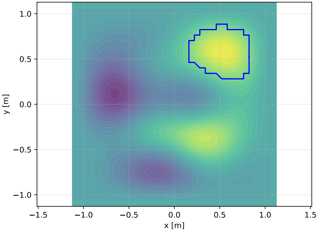
Face 2: xy-plane - Contour 17
