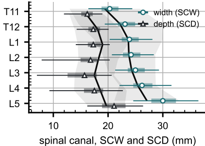
(b) Canal (SCW, SCD)
