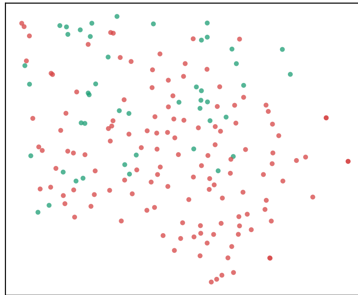
perplejidad=15 · semilla=42
