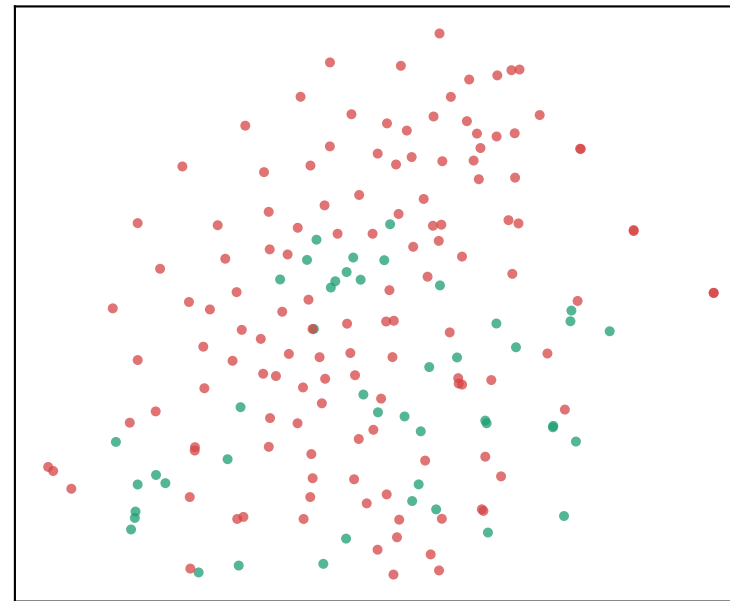
perplejidad=30 · semilla=42
