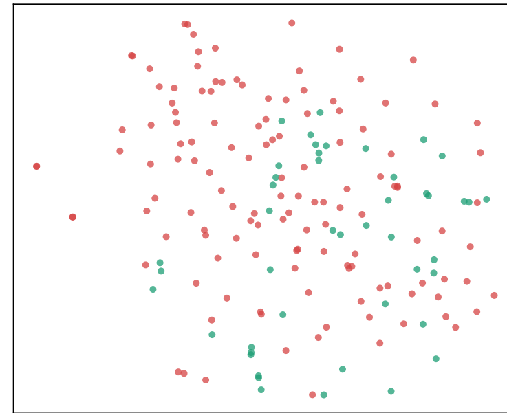
perplejidad=50 · semilla=42
