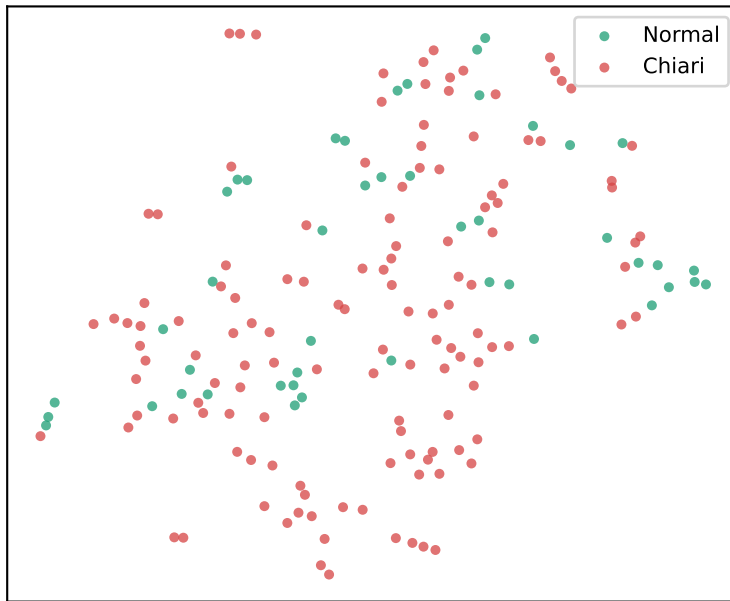
perplejidad=5 · semilla=42
