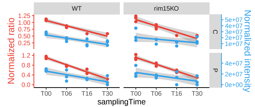
IKI3
