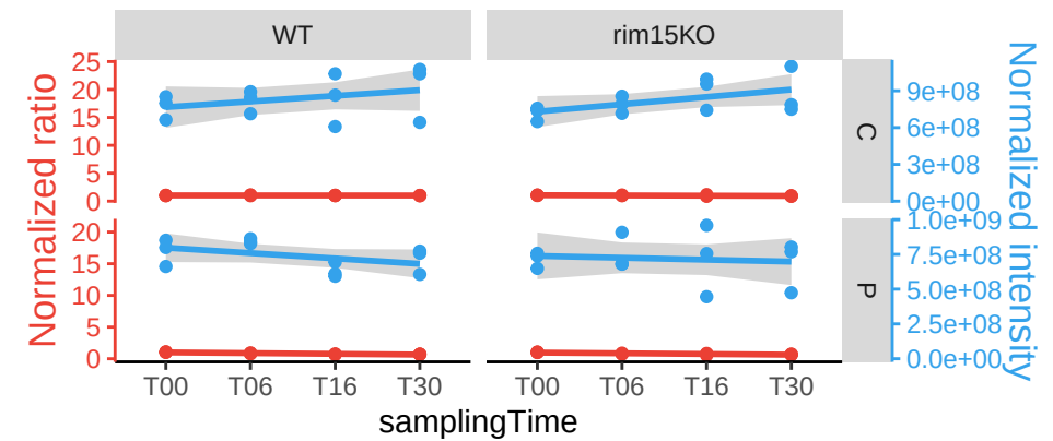
PRE3
