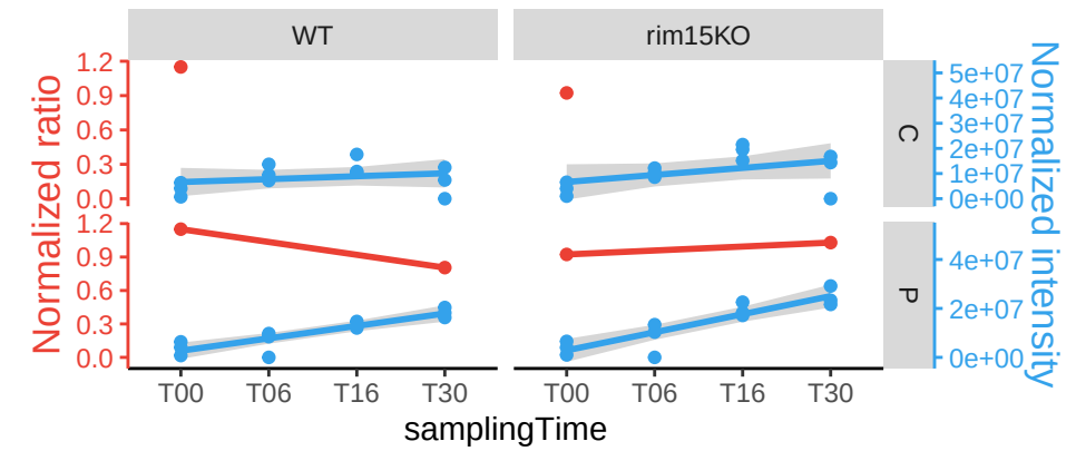
CFT1
