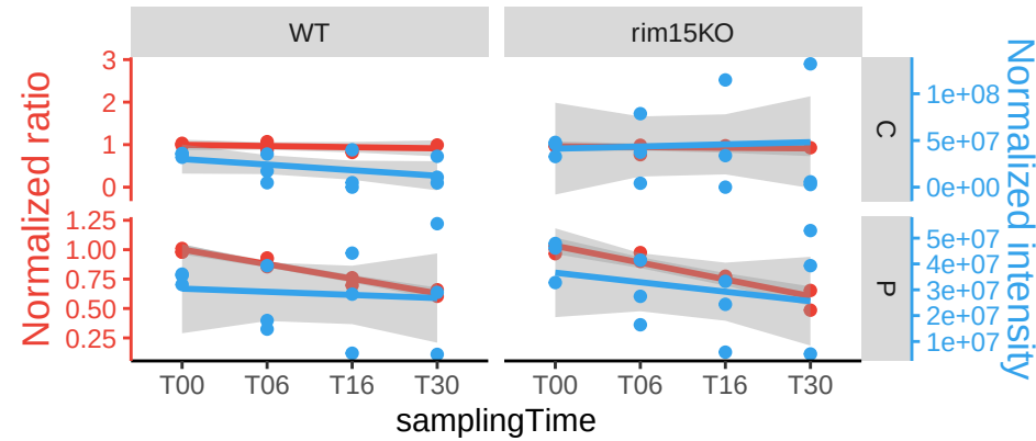
FPK1
