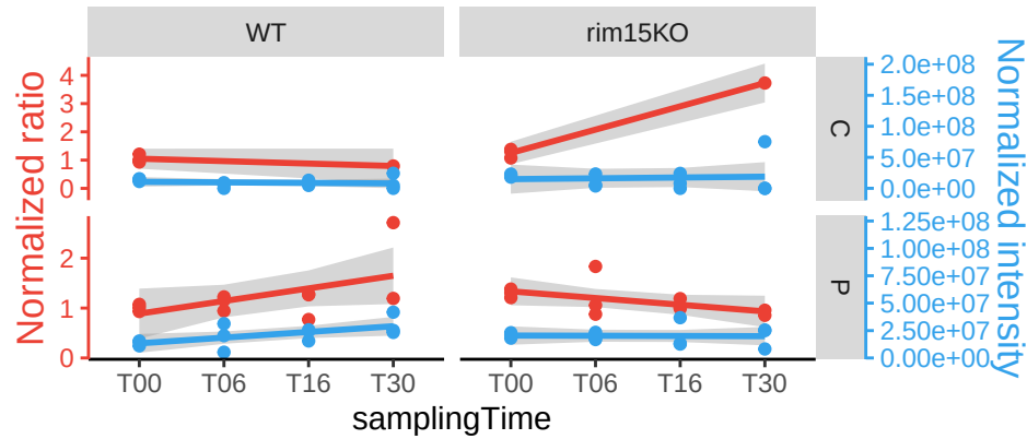
YLR419W
