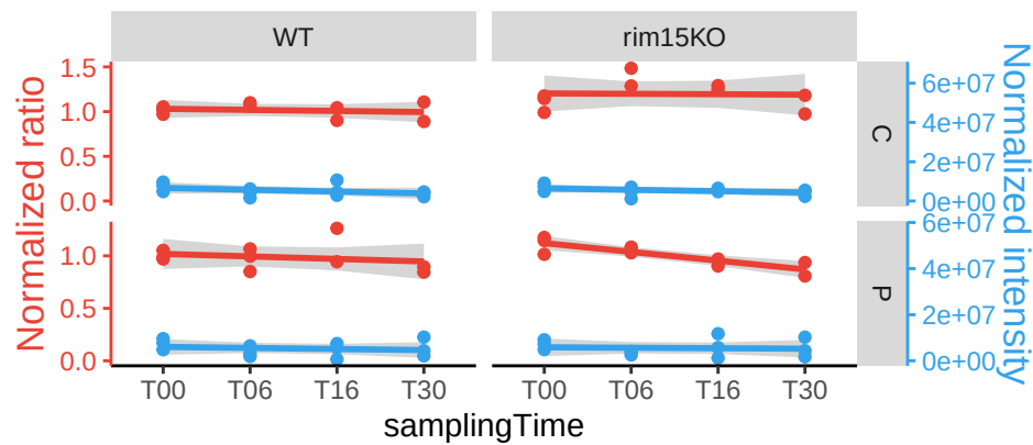
EXO84
