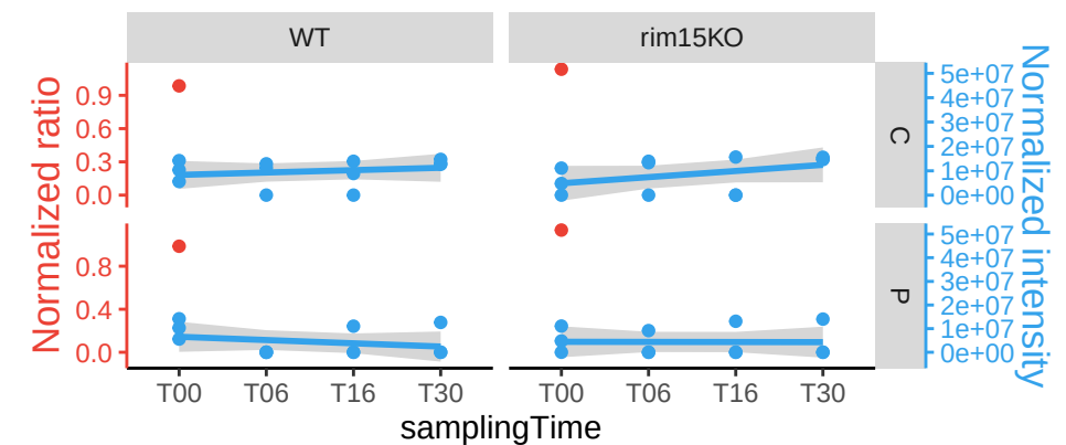
SNX4
