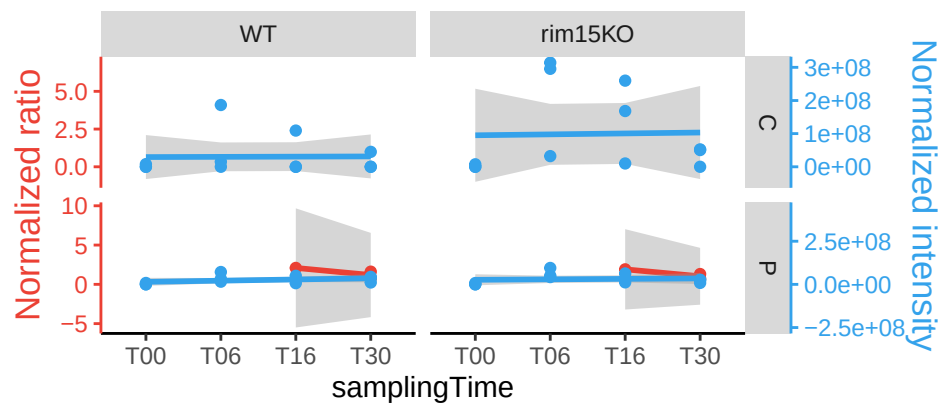
ZUO1
