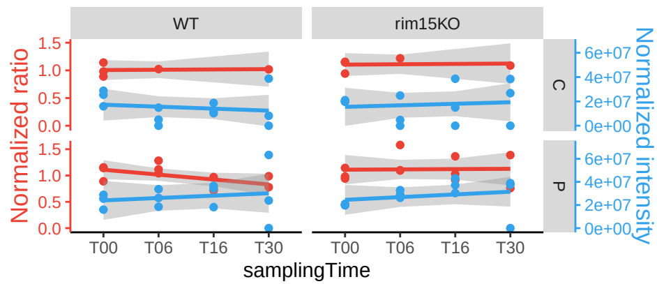
PUF4
