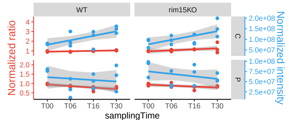
NDC1
