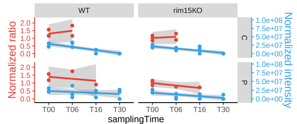
RPF1
