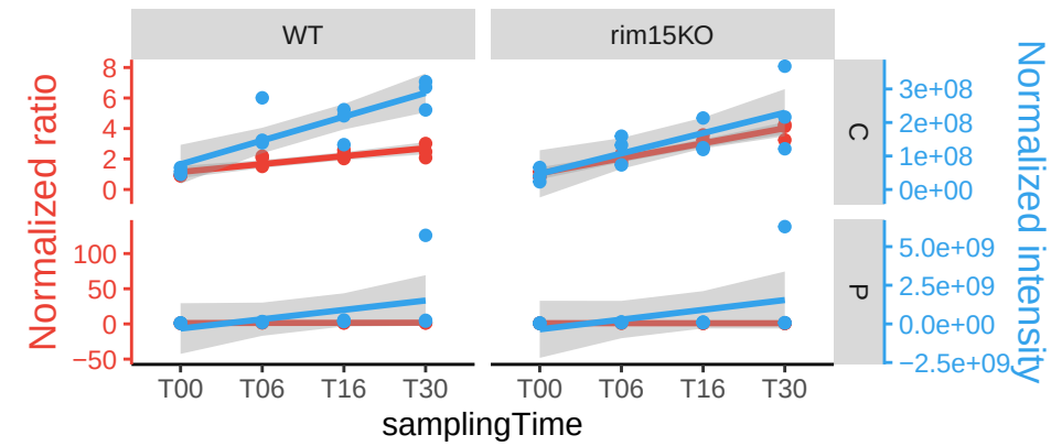
EIS1
