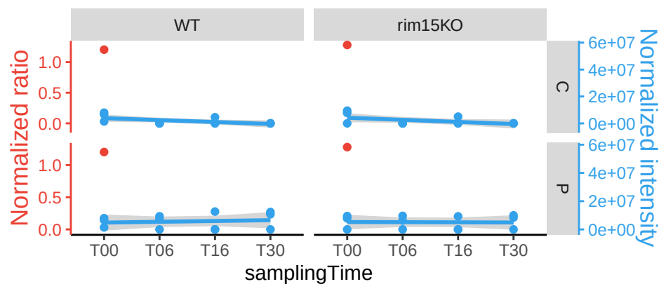
WHI3
