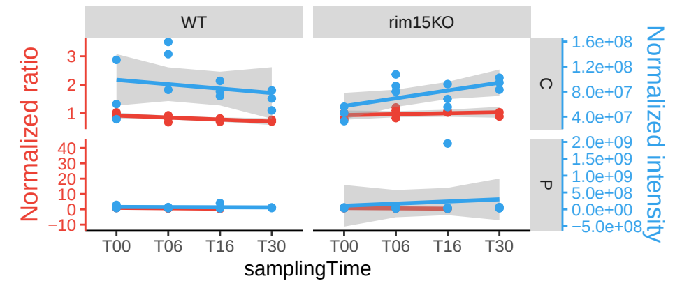
ALG12
