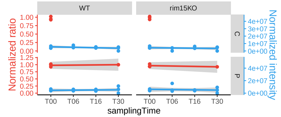
ENP2
