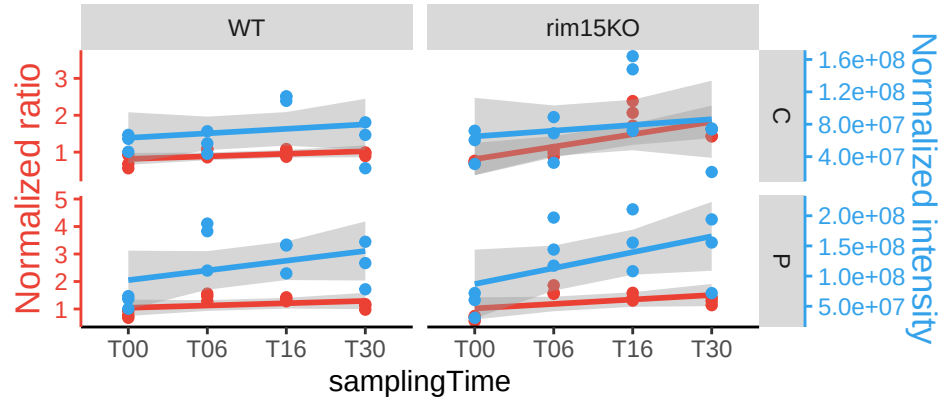
ASP1
