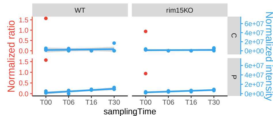
RAV1
