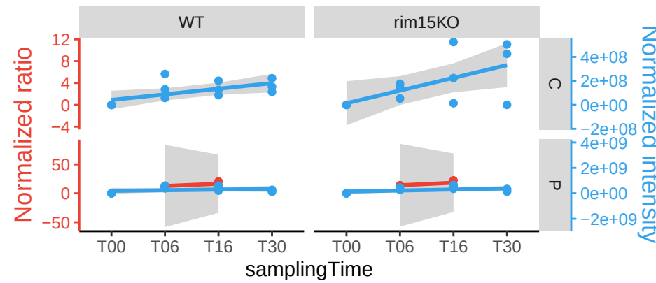
MET3
