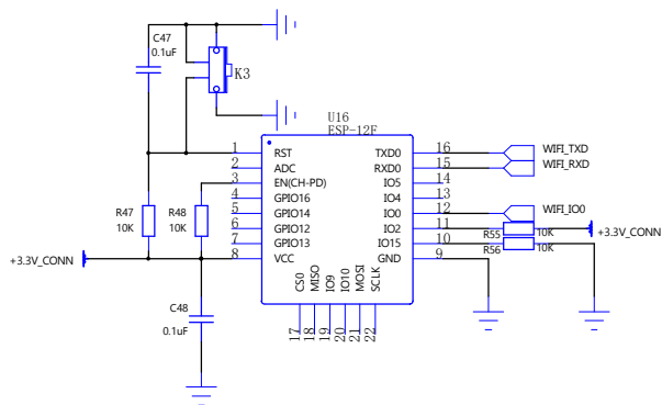
WIFI模块
