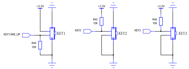
按键
