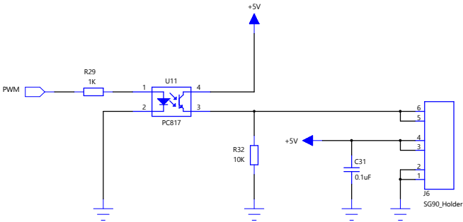
舵机
