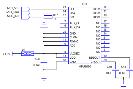
陀螺仪
