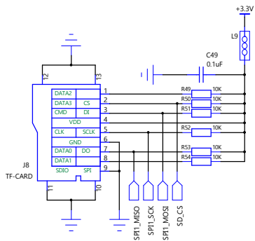
TF卡
