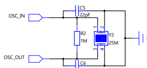
主频时钟
