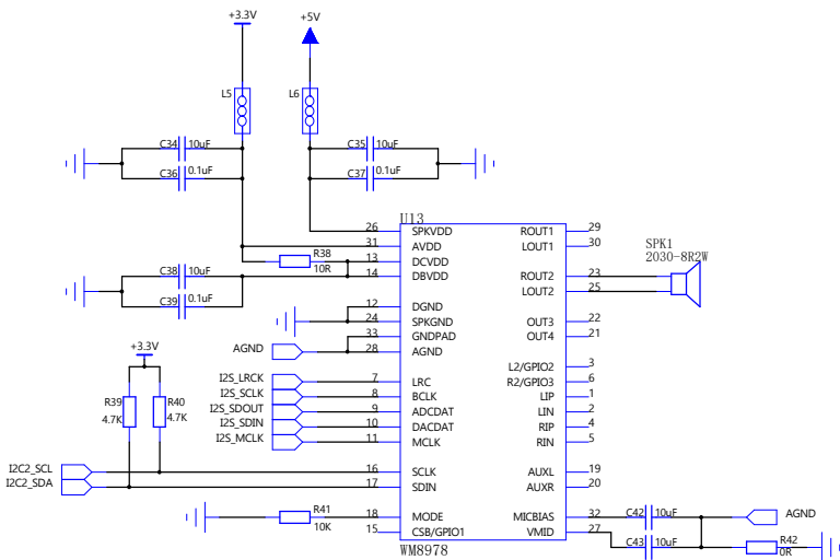
音频解码器
