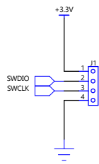
下载调试
