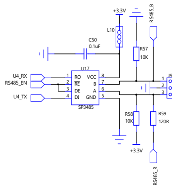
RS485通信
