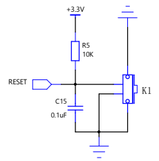
复位电路
