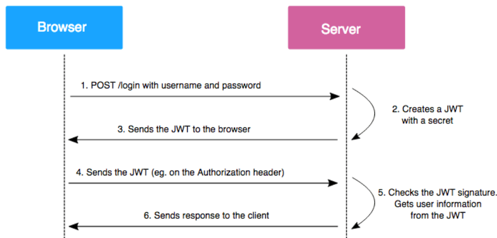
Figura 4.4: Fluxul de autentificare și propagare a tokenului JWT (Tabelul A.1).
