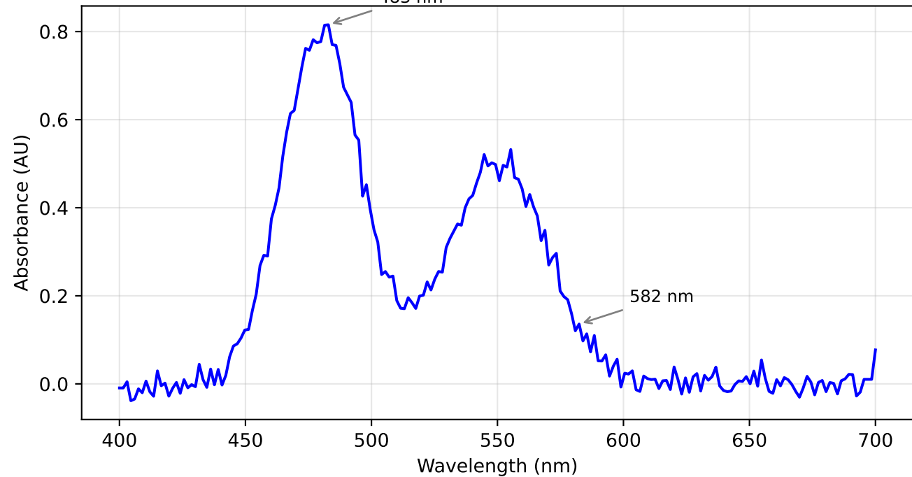
UV-Vis Spectrum
