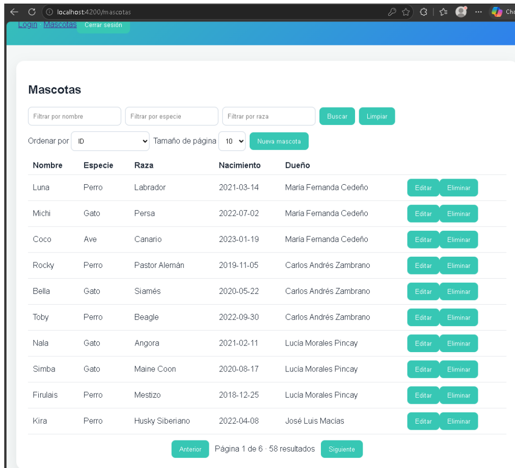
Figura 6: Listado de mascotas registradas en BIOPET.
