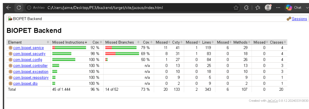
Figura 15: Reporte de cobertura de JaCoCo, con 99.42 % de líneas y 73.08 % de ramas cubiertas.
