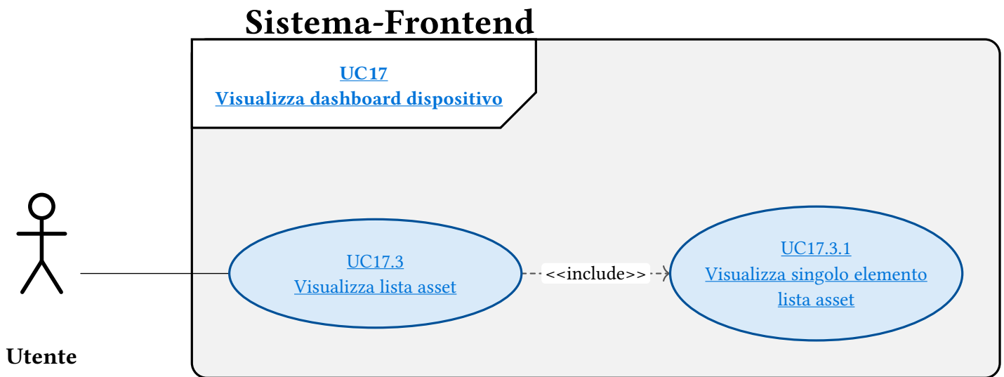
Figura 21: UC17.3 - Visualizza lista asset
