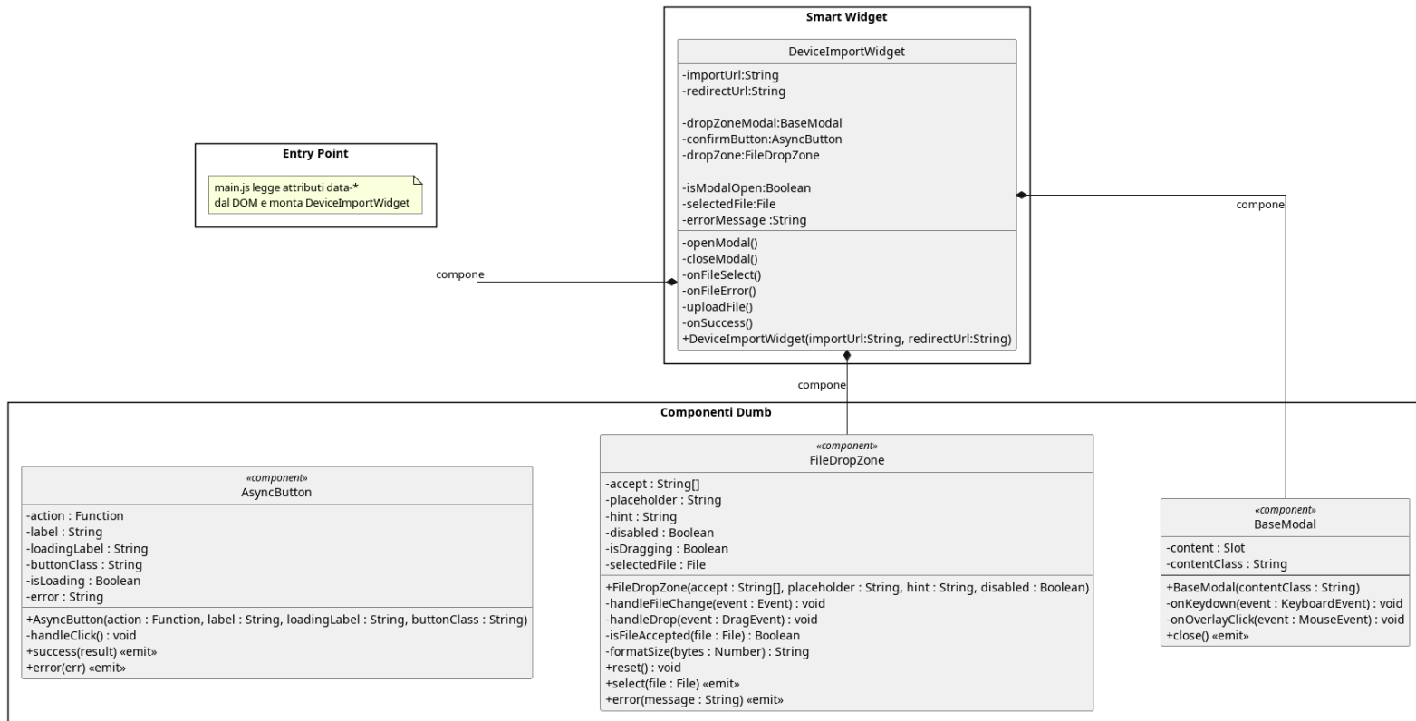
Figura 182: DeviceImport
