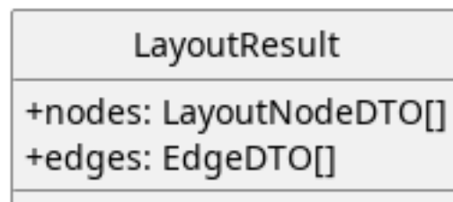
Figura 206: LayoutResult
