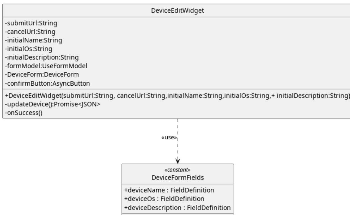
Figura 179: Widget - DeviceEditWidget
