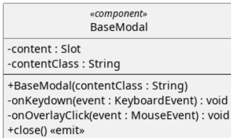
Figura 164: Componente - BaseModal
