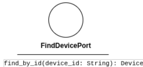
Figura 48: FindDevicePort
