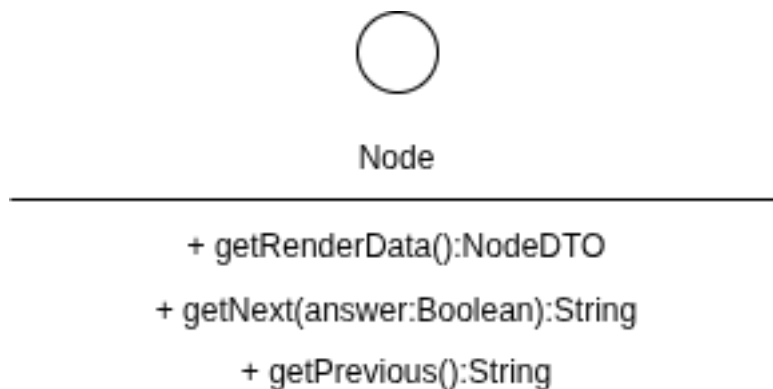
Figura 193: Node
