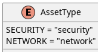
Figura 10: AssetType
