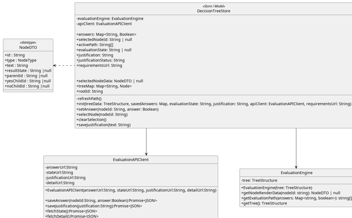
Figura 209: DecisionTreeComplessivo
