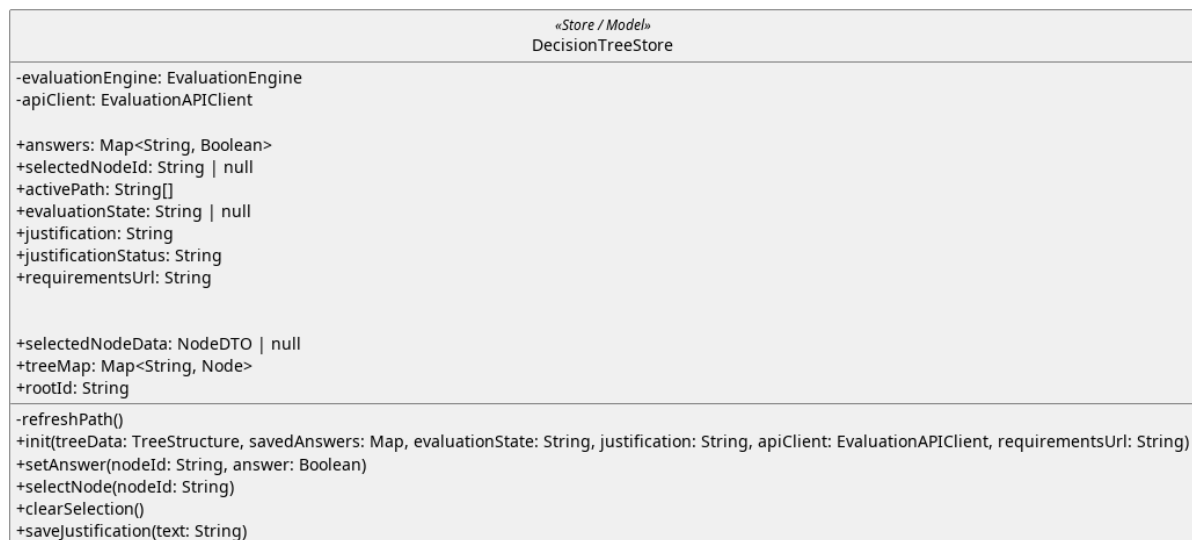
Figura 210: DecisionTreeStore
