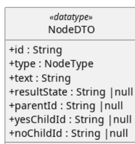
Figura 197: NodeDTO
