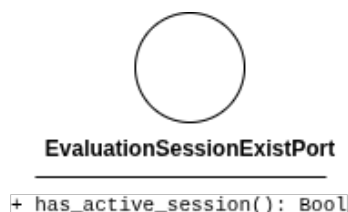
Figura 131: EvaluationSessionExistPort
