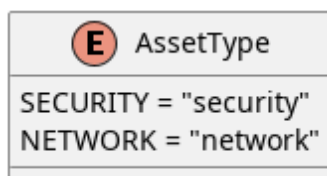
Figura 9: AssetType
