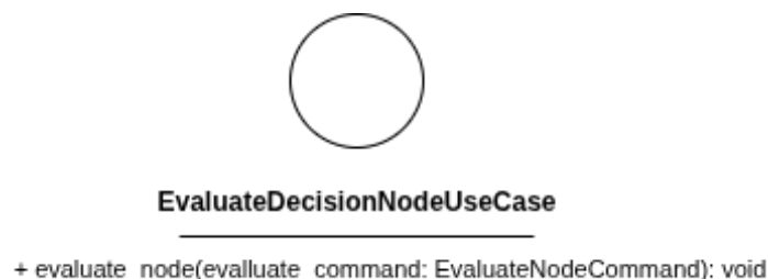
Figura 144: EvaluateDecisionNodeUseCase
