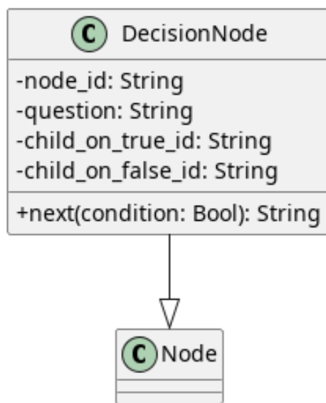
Figura 15: DecisionNode
