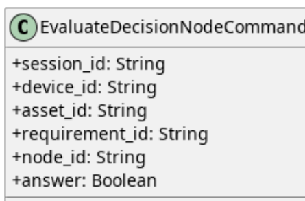
Figura 145: EvaluateDecisionNodeCommand
