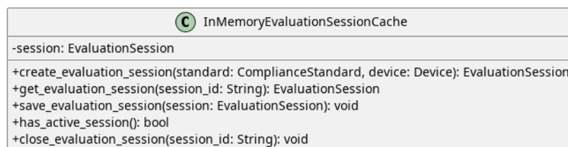
Figura 75: InMemoryEvaluationSessionCache
