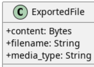
Figura 29: ExportedFile
