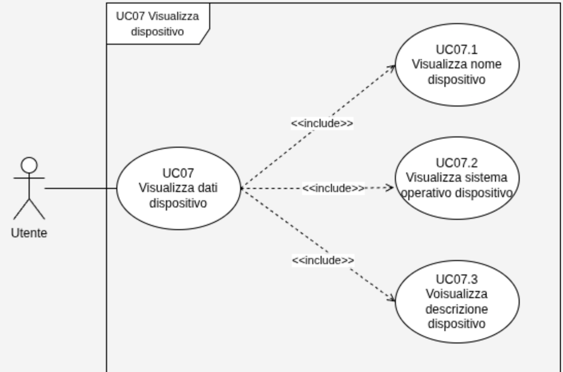
Sistema - Frontend
