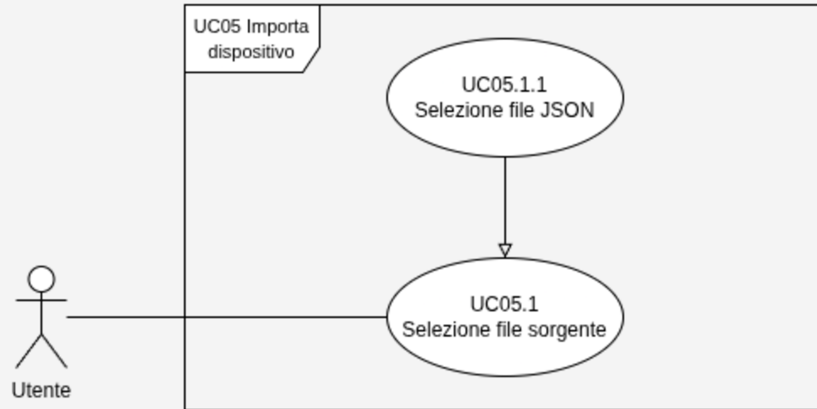
Sistema - Frontend
