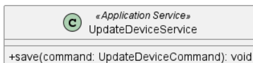
Figura 20: UpdateDeviceService
