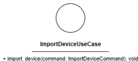
Figura 64: ImportDeviceUseCase
