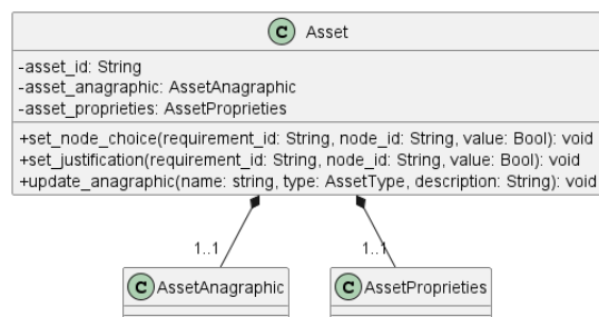
Figura 39: Asset
