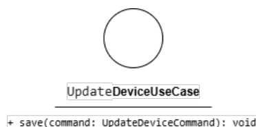
Figura 18: UpdateDeviceUseCase
