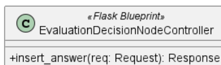
Figura 118: EvaluationDecisionNodeController
