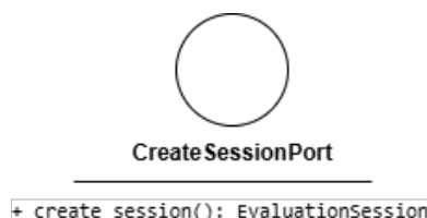
Figura 97: CreateSessionPort
