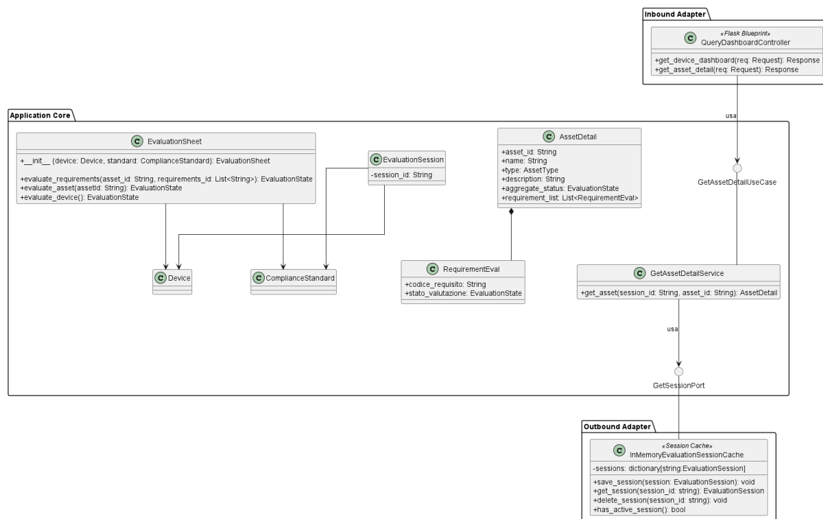
Figura 51: Diagramma delle classi — Caso d'uso GetAssetDetail
