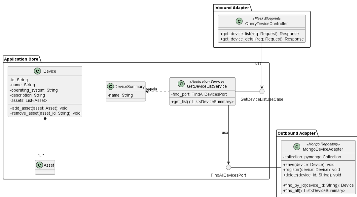
Figura 28: Caso d'uso GetDeviceList
