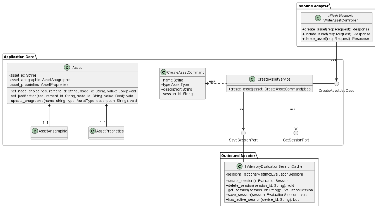
Figura 33: Caso d'uso CreateAsset
