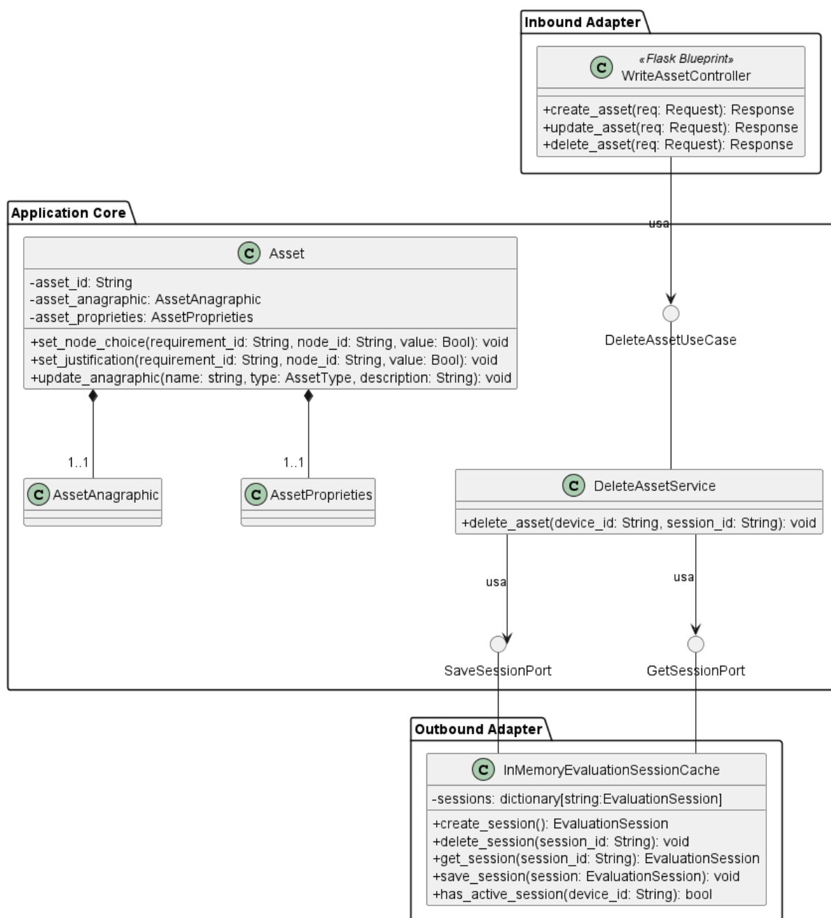
Figura 48: Caso d'uso DeleteAsset
