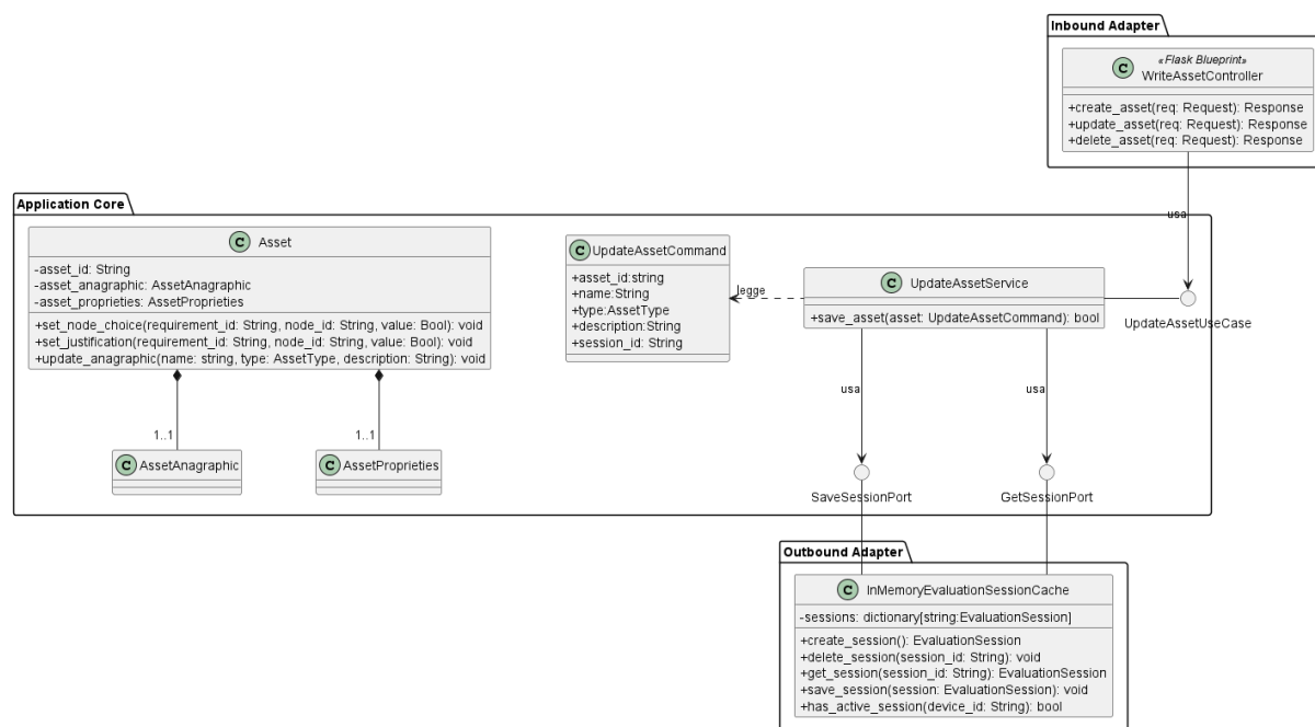
Figura 44: Caso d'uso UpdateAsset
