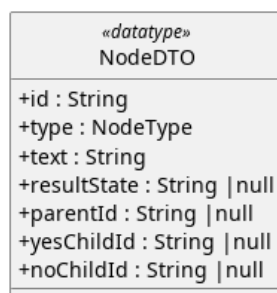
Figura 196: NodeDTO
