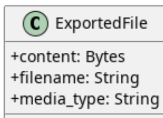
Figura 29: ExportedFile
