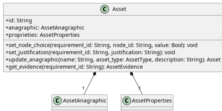
Figura 6: Asset
