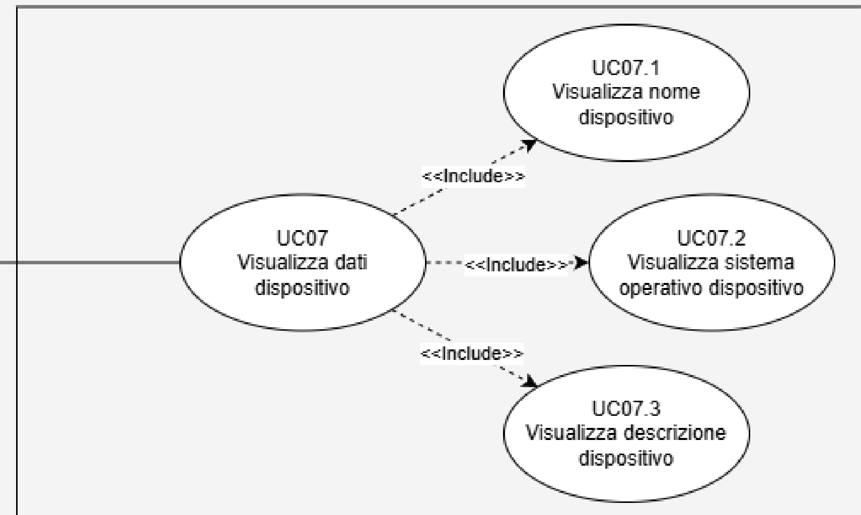
Sistema-Frontend
