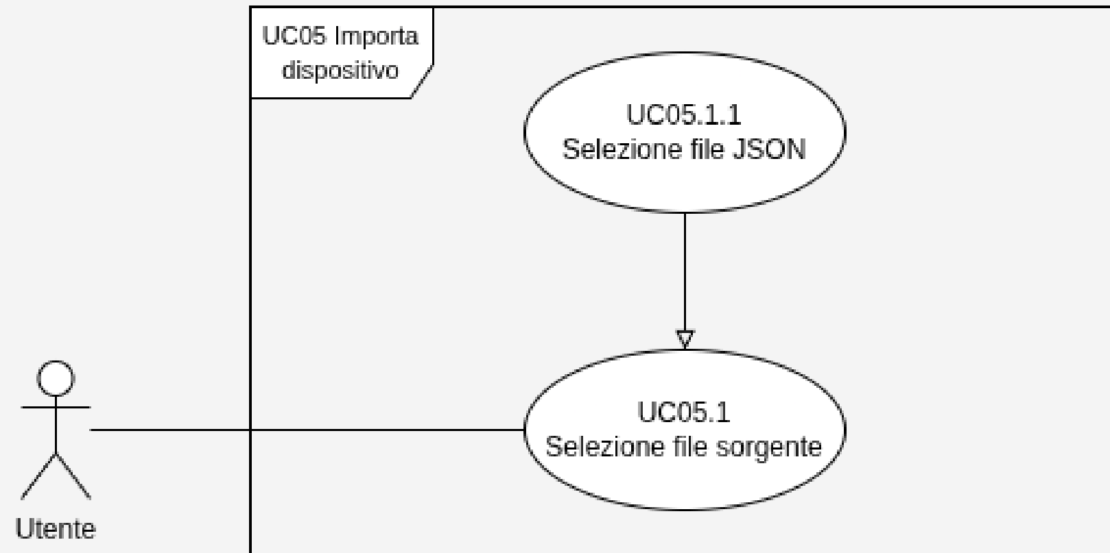
Utente
