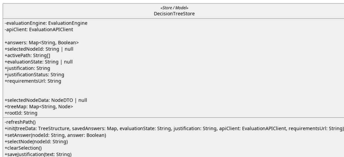
Figura 210: DecisionTreeStore
