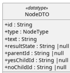
Figura 196: NodeDTO
