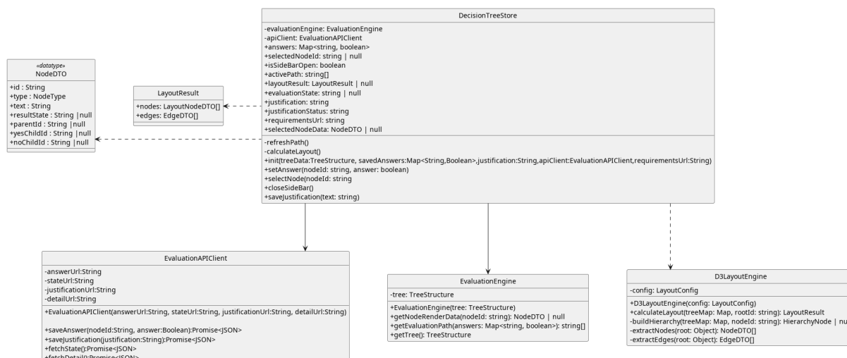
Figura 208: DecisionTreeComplessivo
