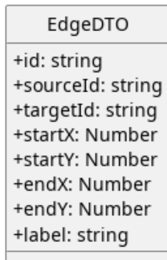
Figura 203: EdgeDTO
