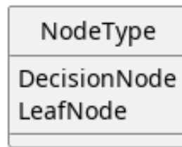
Figura 197: NodeType
