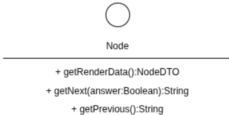
Figura 193: Node
