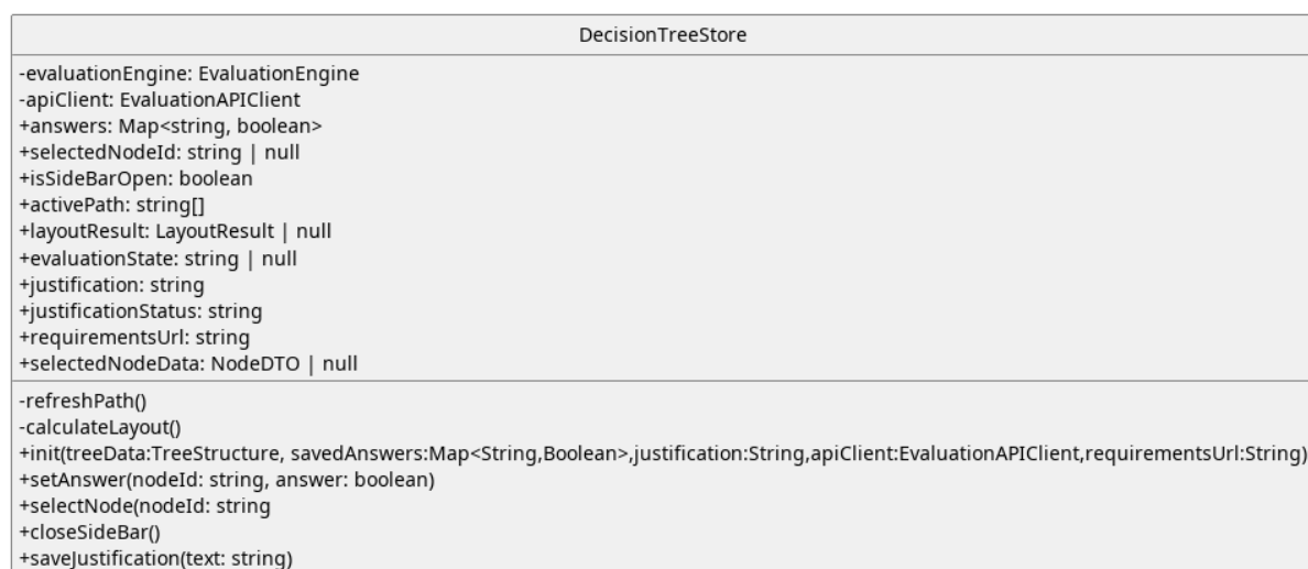
Figura 209: DecisionTreeStore
