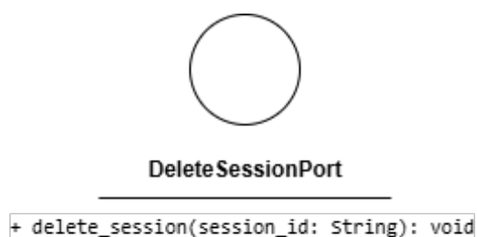
Figura 148: DeleteSessionPort
