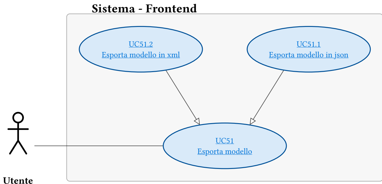
Figura 92: UC51 - Esporta modello
