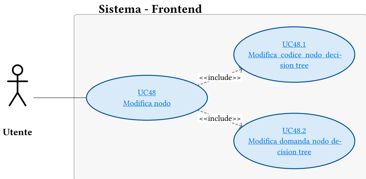
Figura 88: UC48 - Modifica nodo
