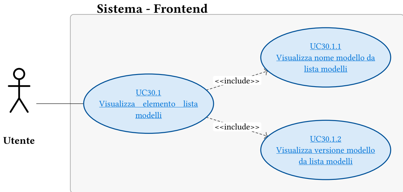
Figura 49: UC30.1 - Visualizza elemento lista modelli
