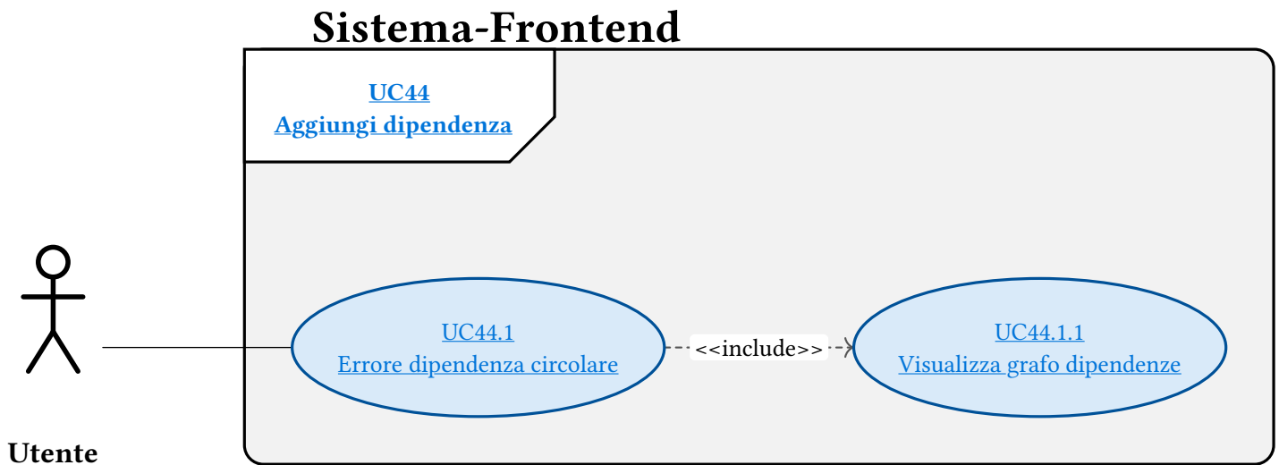
Figura 80: UC44.1 - Errore dipendenza circolare
