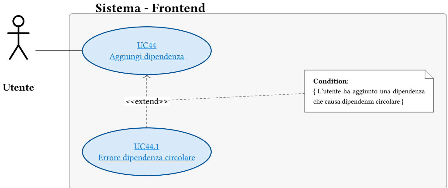
Figura 79: UC44 - Aggiungi dipendenza
