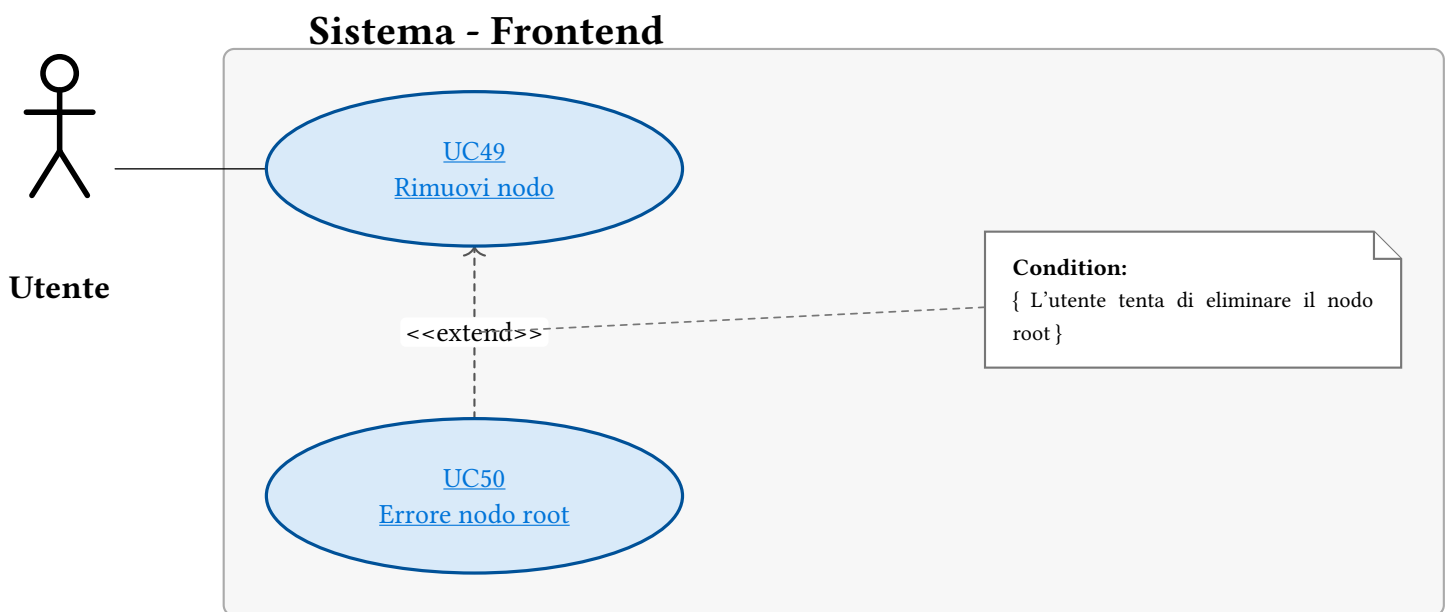
Figura 91: UC49 - Rimuovi nodo
