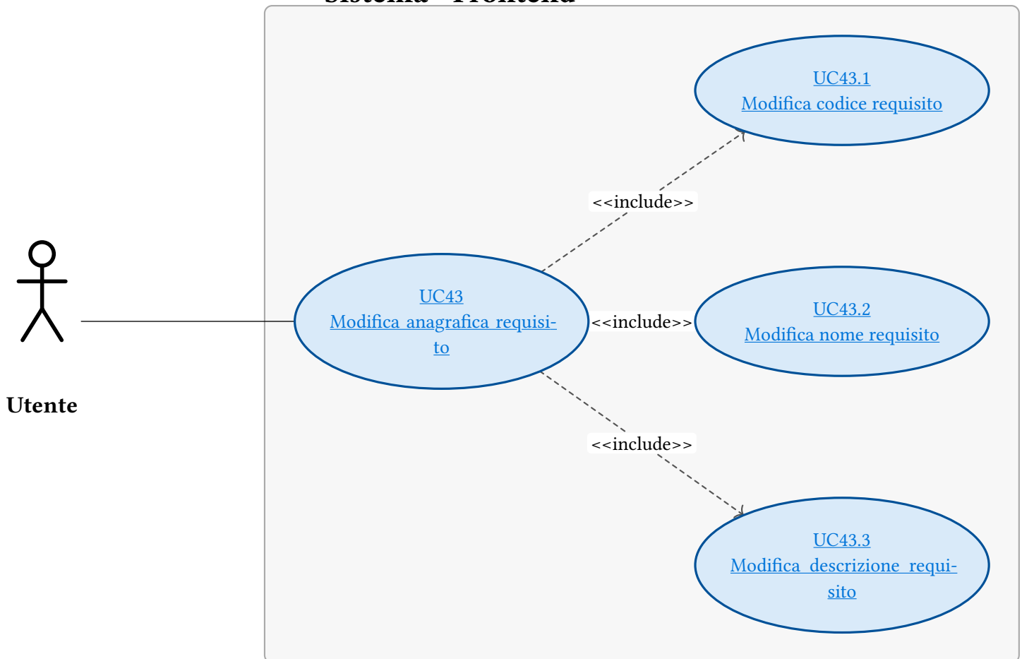
Figura 76: UC43 - Modifica anagrafica requisito
