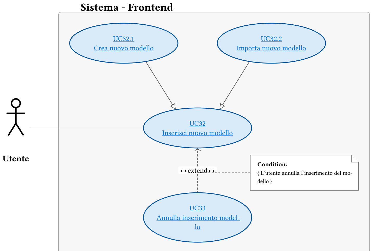
Figura 53: UC32 - Inserisci nuovo modello
