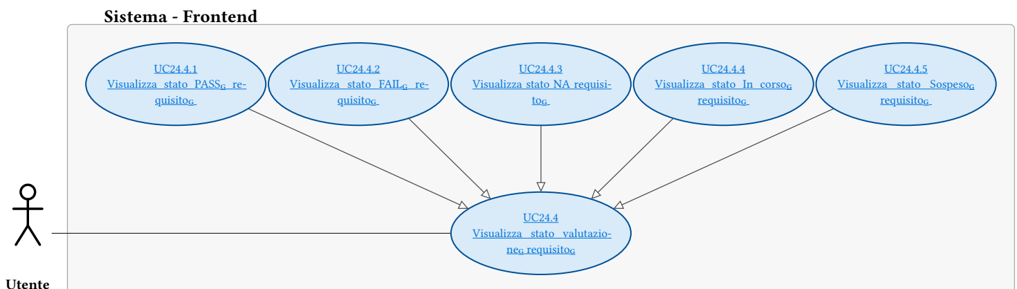
Figura 33: UC24.4 - Visualizza stato valutazione G requisito G
