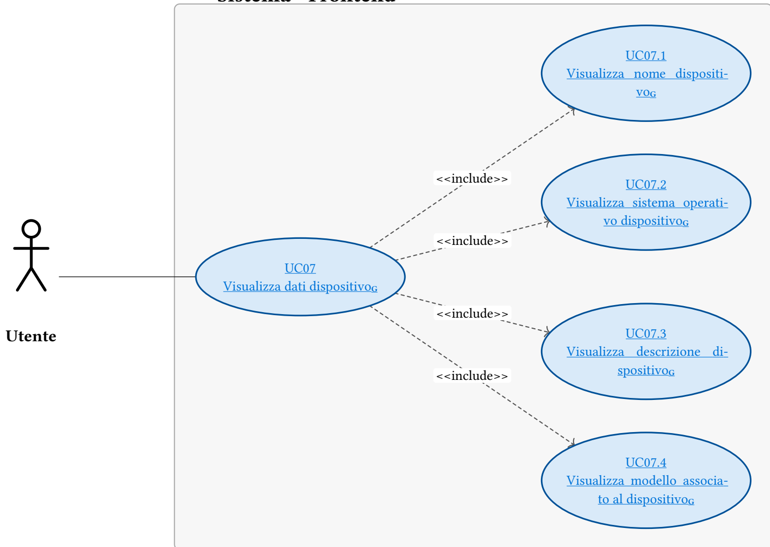
Figura 8: UC07 - Visualizza dati dispositivo G
