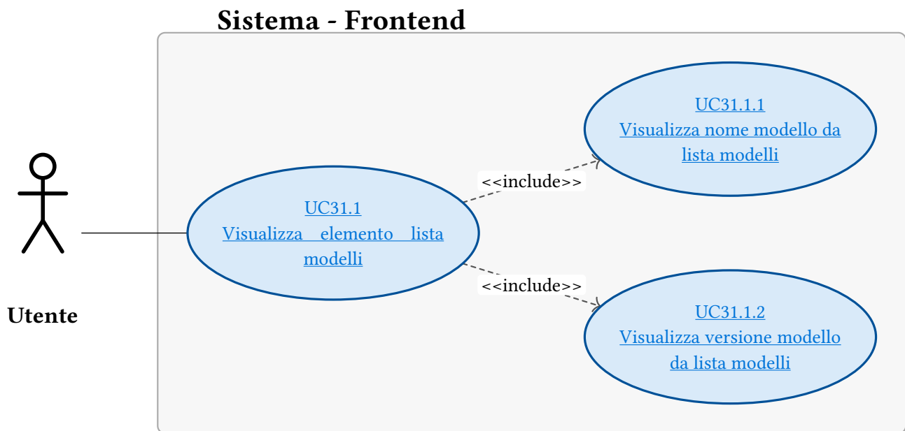
Figura 49: UC31.1 - Visualizza elemento lista modelli
