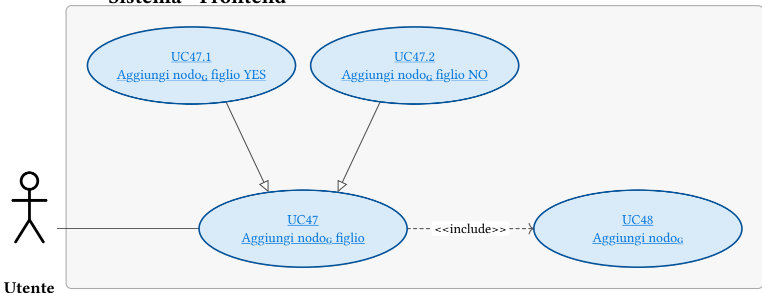
Figura 82: UC47 - Aggiungi nodo G figlio
