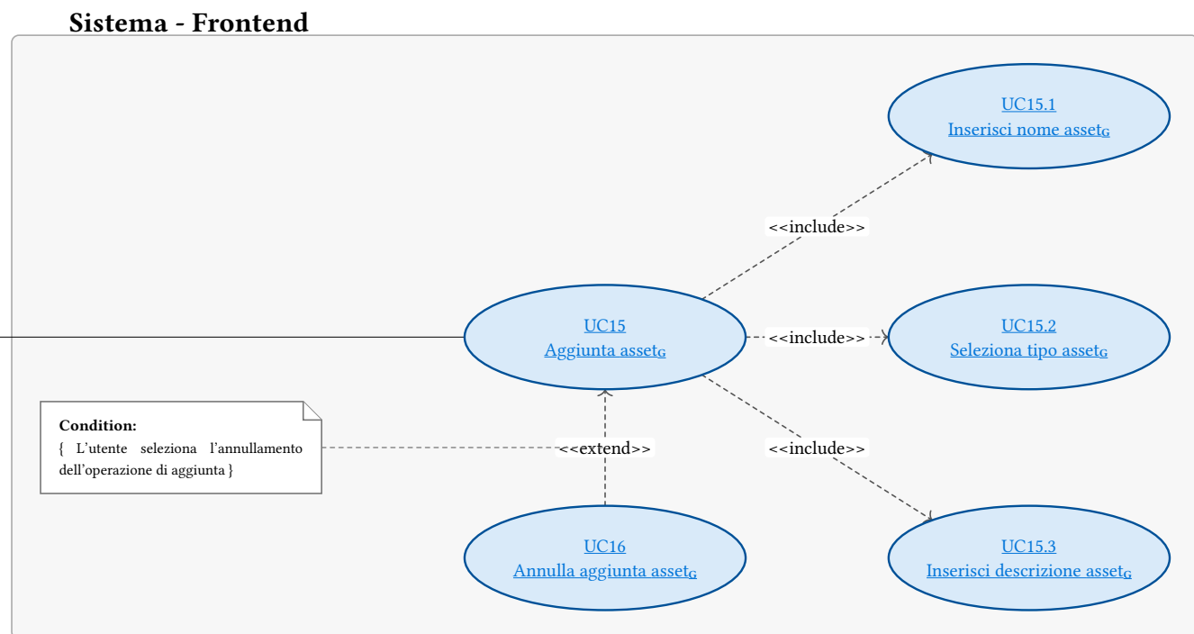
Figura 16: UC15 - Aggiunta asset G
