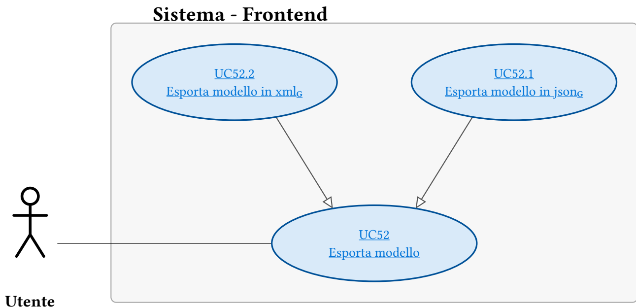
Figura 92: UC52 - Esporta modello
