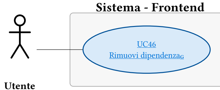
Figura 81: UC46 - Rimuovi dipendenza G
