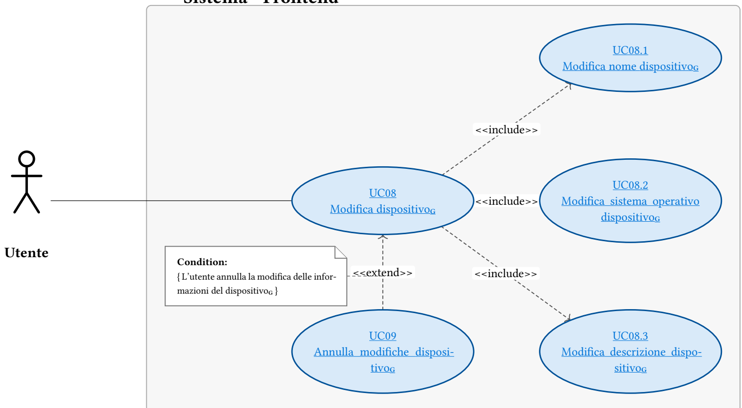
Figura 10: UC08 - Modifica dispositivo G
