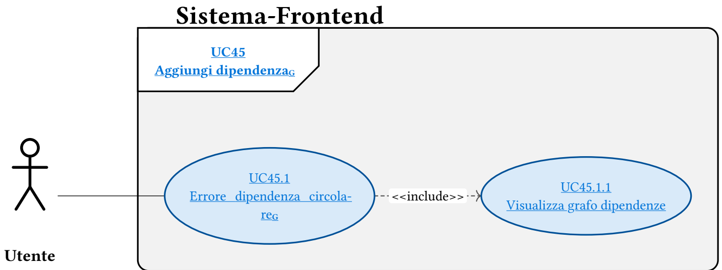
Figura 80: UC45.1 - Errore dipendenza circolare G
