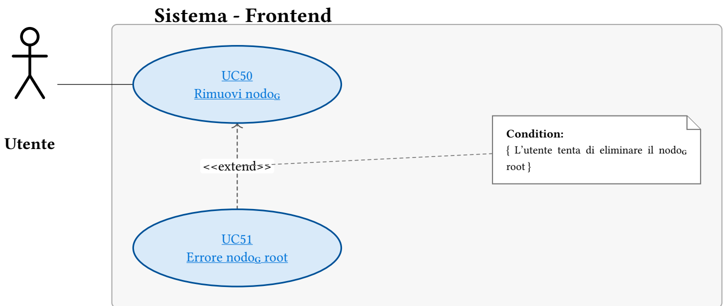
Figura 91: UC50 - Rimuovi nodo G
