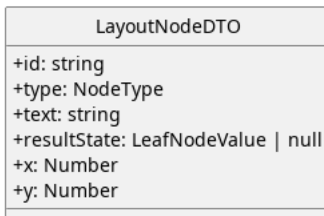
Figura 203: LayoutNodeDTO
