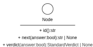
Figura 15: Node
