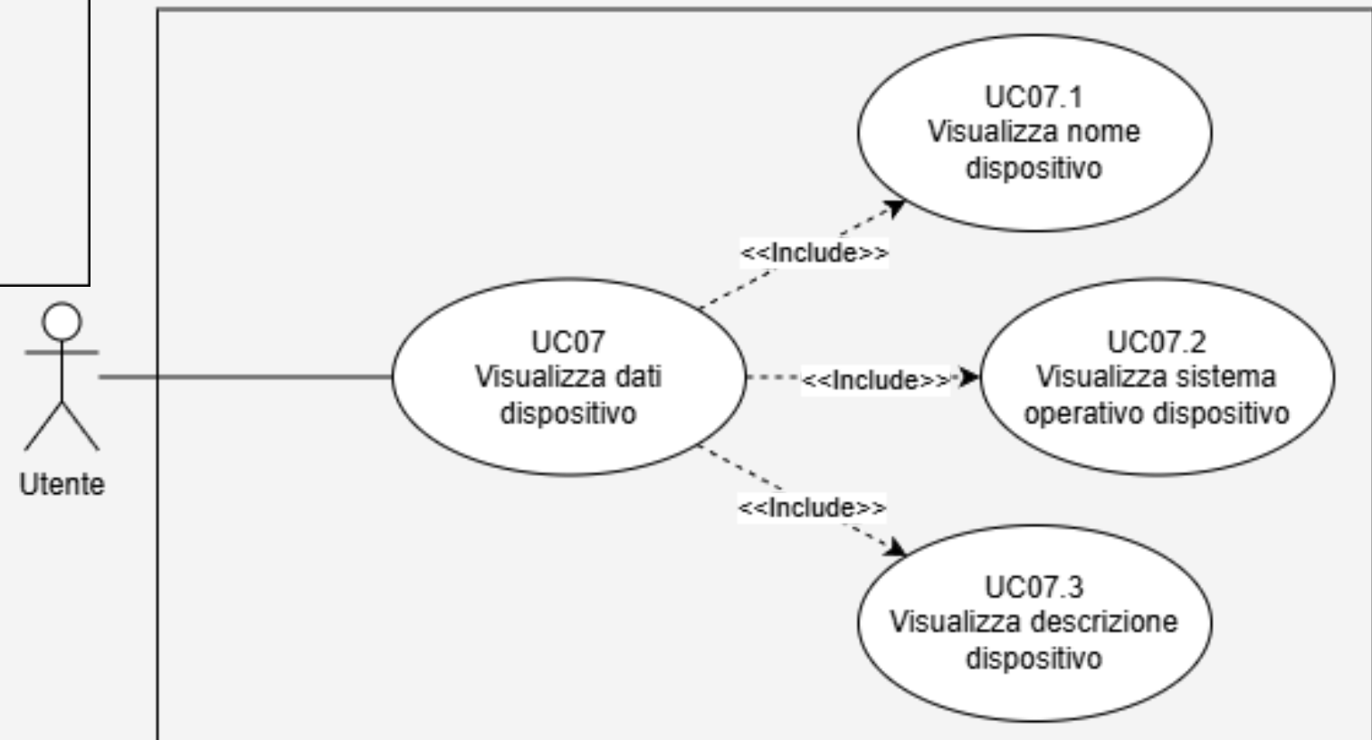
Sistema-Frontend
