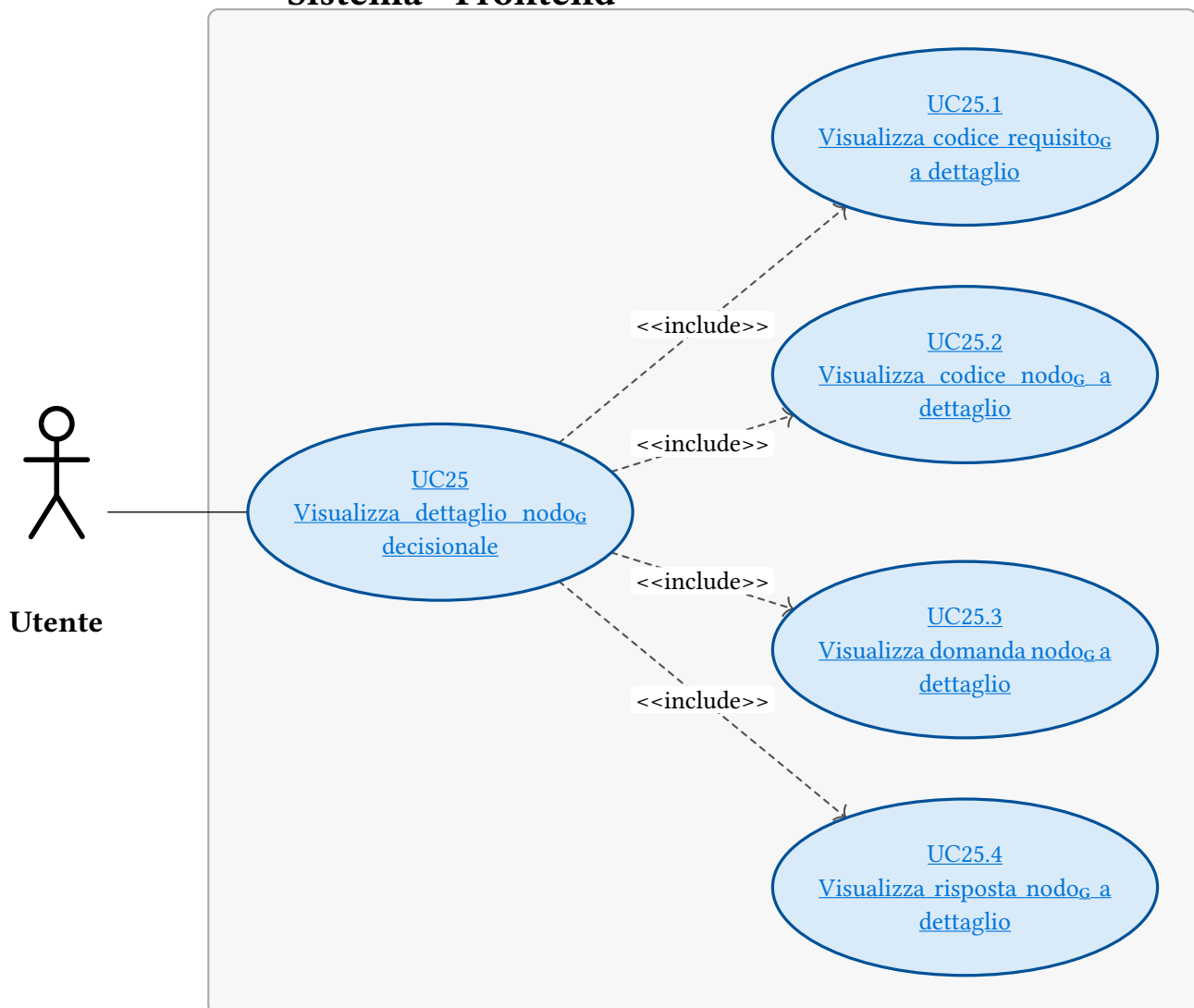
Figura 41: UC25 - Visualizza dettaglio nodo C decisionale
