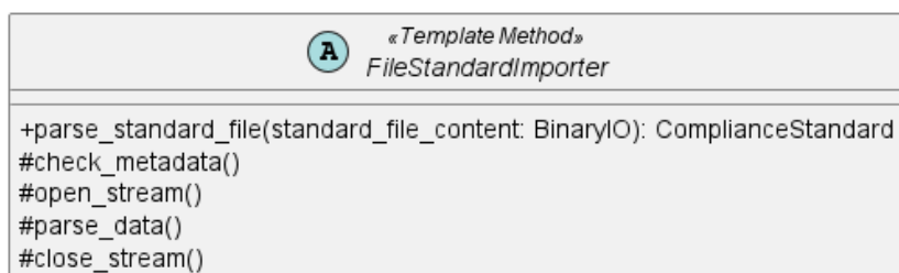
Figura 82: FileStandardImporter
