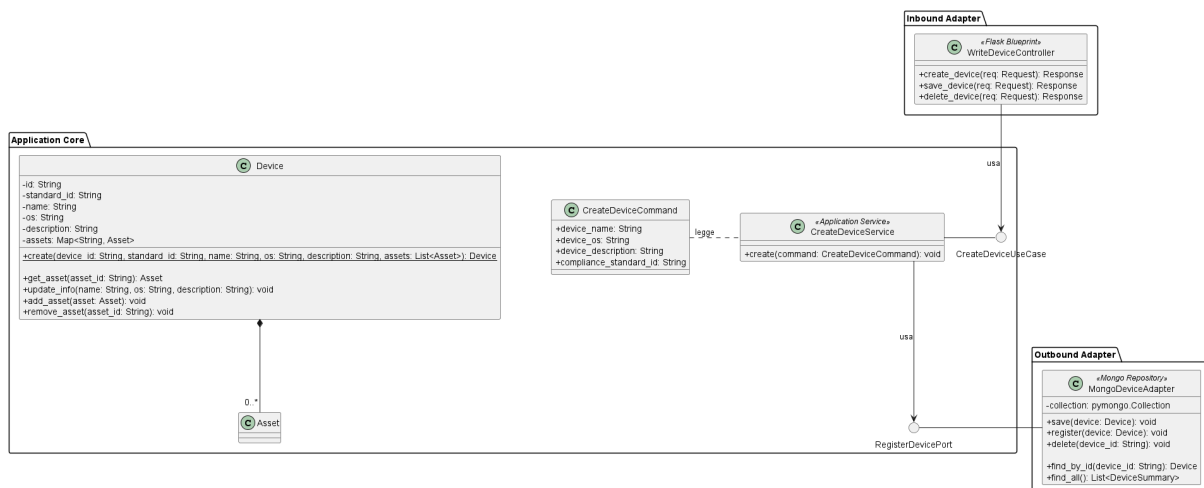
Figura 4: Caso d'uso CreateDevice
