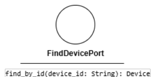
Figura 28: FindDevicePort
