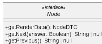
Figura 178: Interfaccia Node
