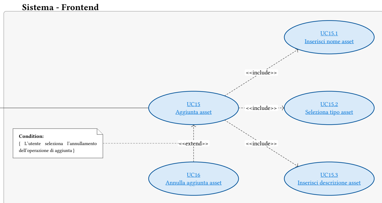
Figura 16: UC15 - Aggiunta asset
