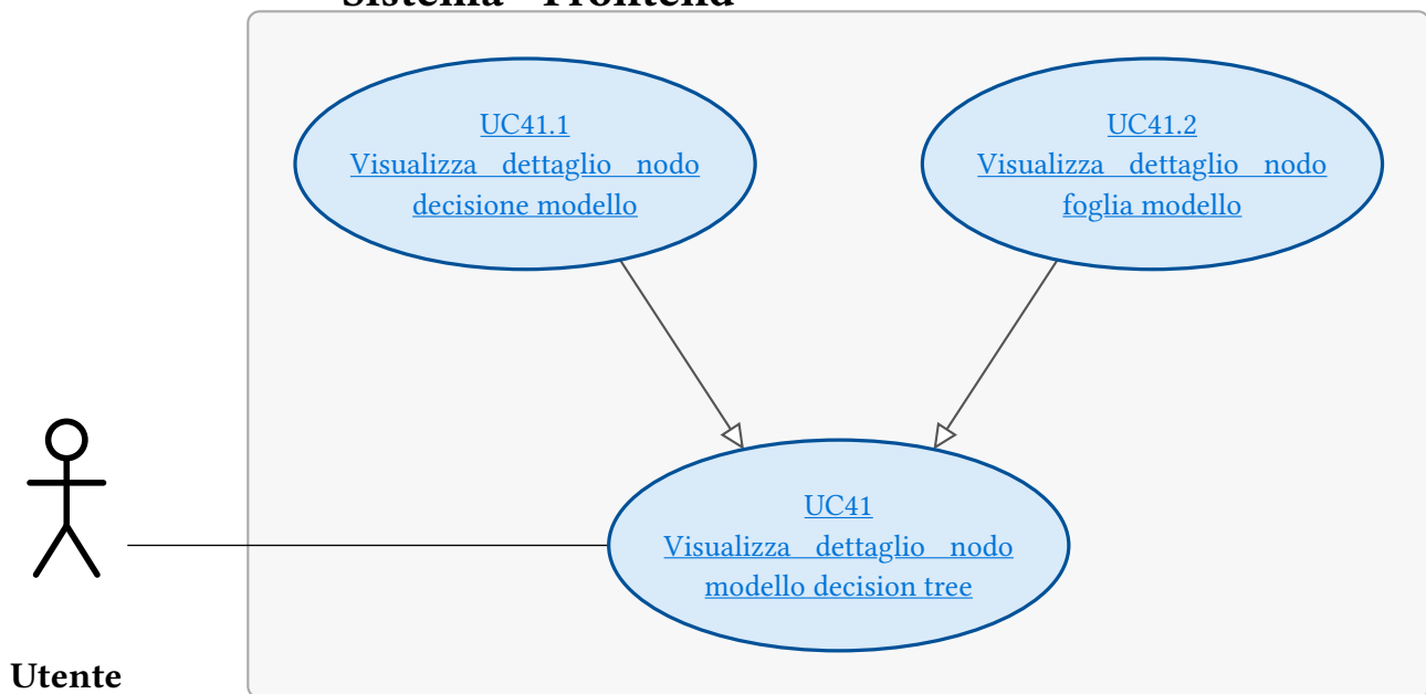
Figura 70: UC41 - Visualizza dettaglio nodo modello decision tree
