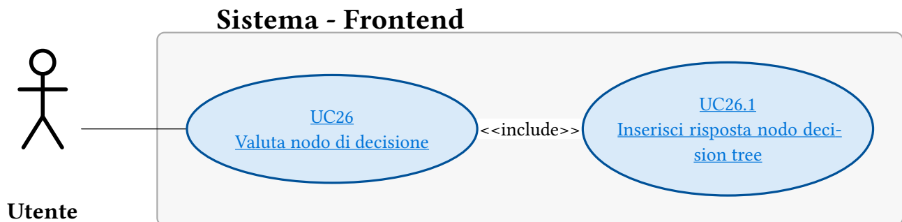
Figura 43: UC26 - Valuta nodo di decisione
