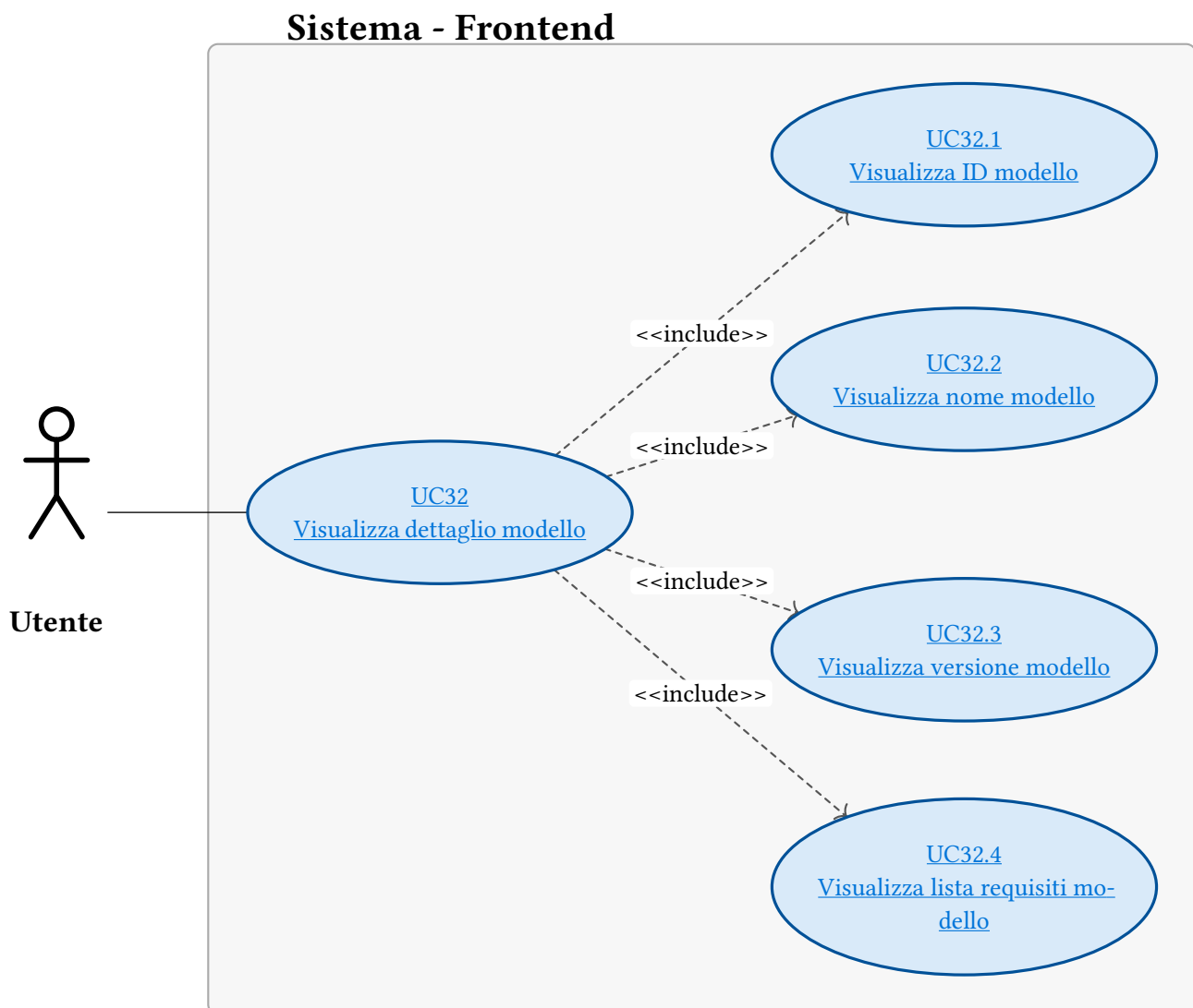
Figura 50: UC32 - Visualizza dettaglio modello
