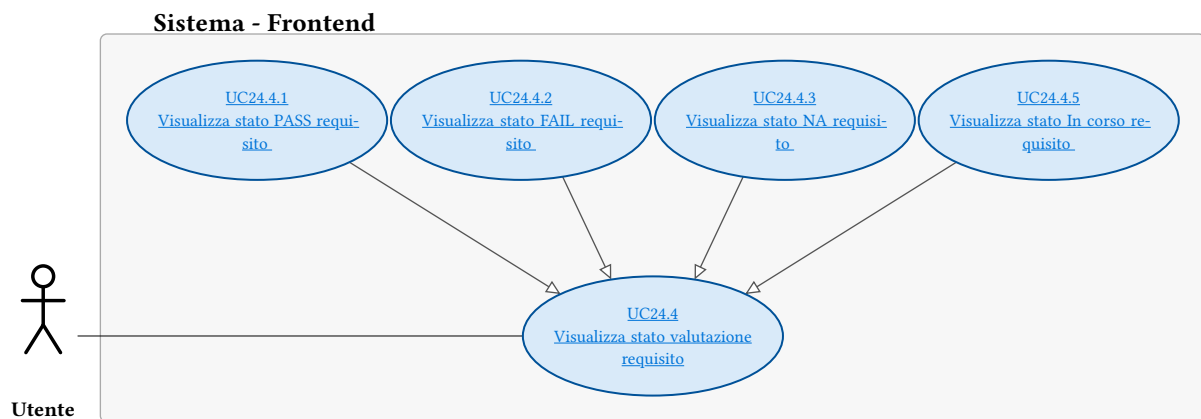
Figura 33: UC24.4 - Visualizza stato valutazione requisito
