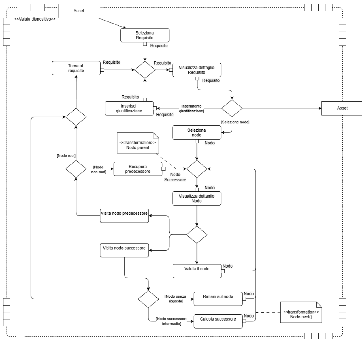
Figura 31: UC23 - Valuta asset
