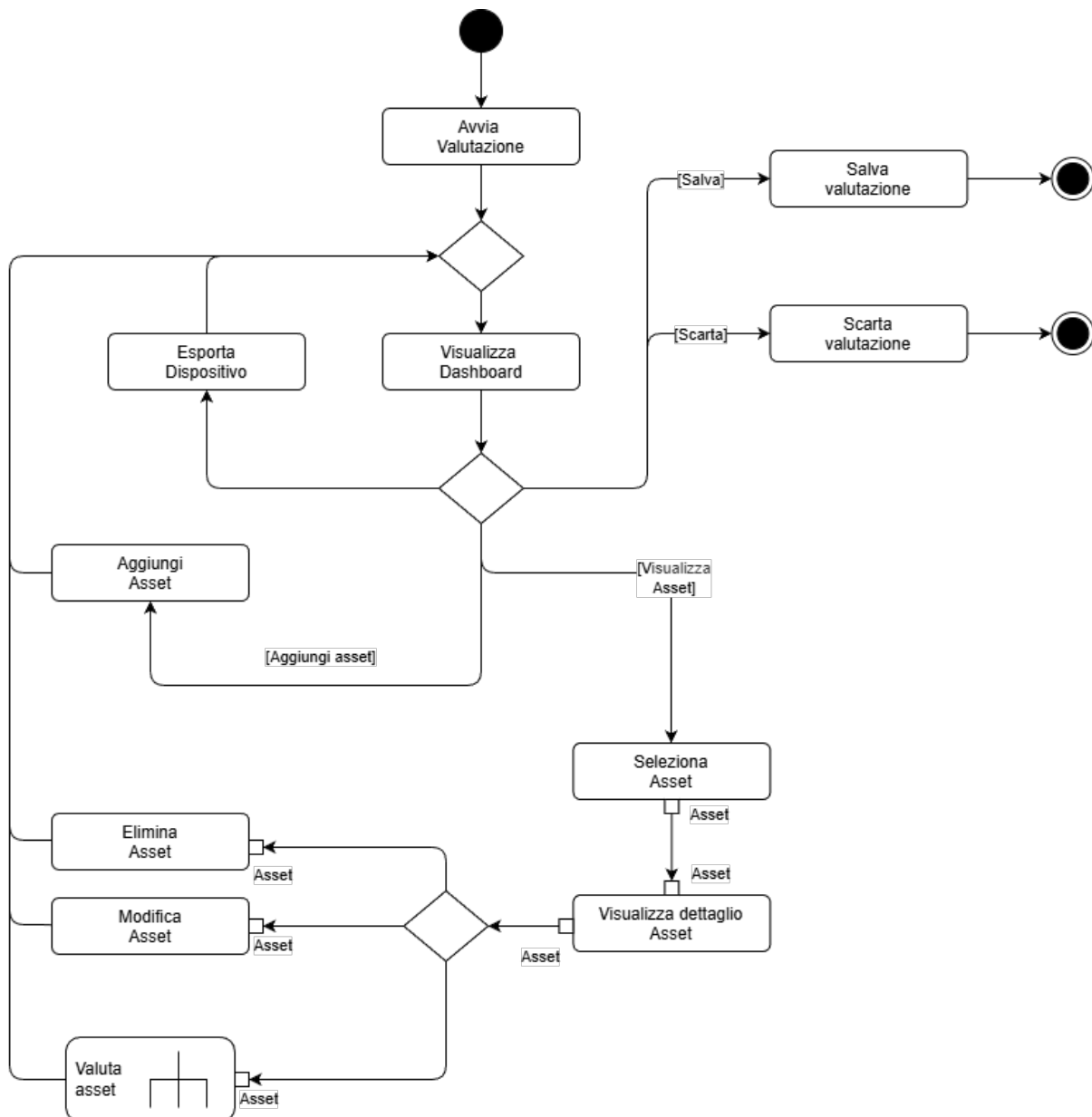
Figura 13: UC11 - Avvia valutazione dispositivo
