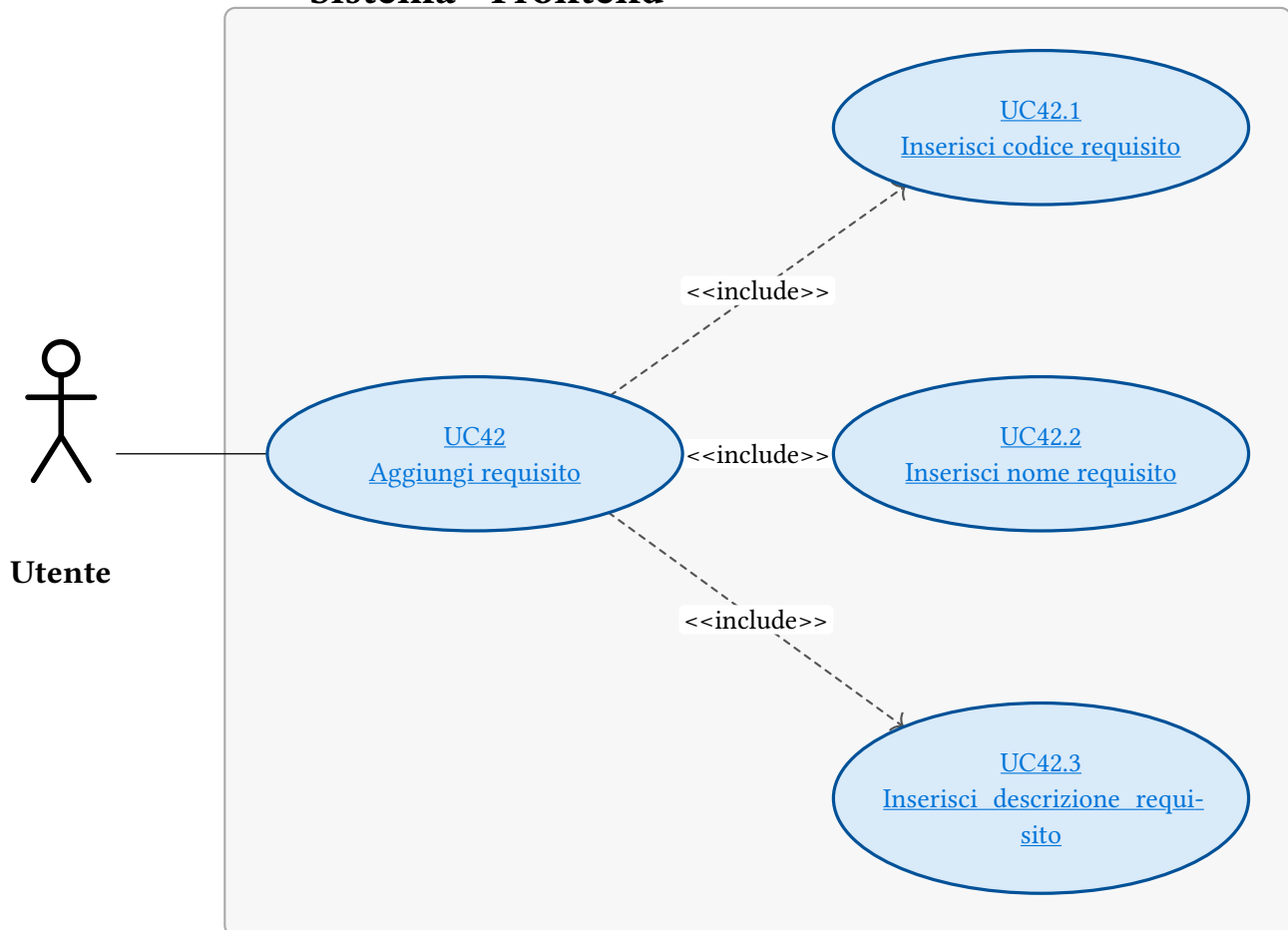
Figura 72: UC42 - Aggiungi requisito
