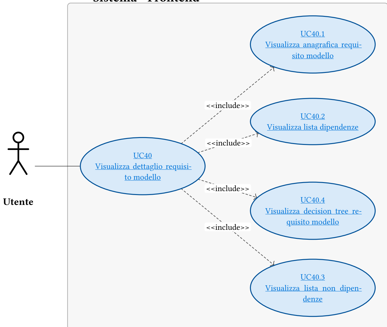
Figura 63: UC40 - Visualizza dettaglio requisito modello
