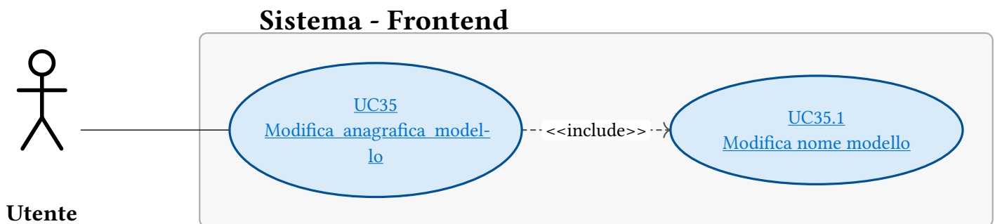
Figura 57: UC35 - Modifica anagrafica modello
