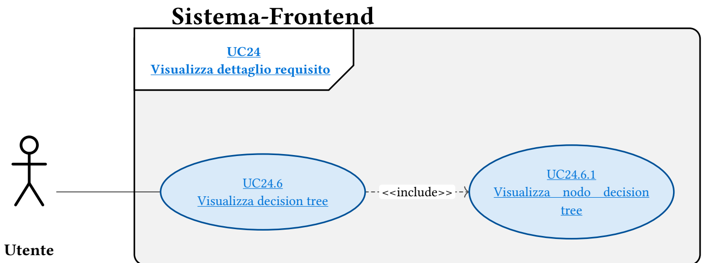
Figura 36: UC24.6 - Visualizza decision tree
