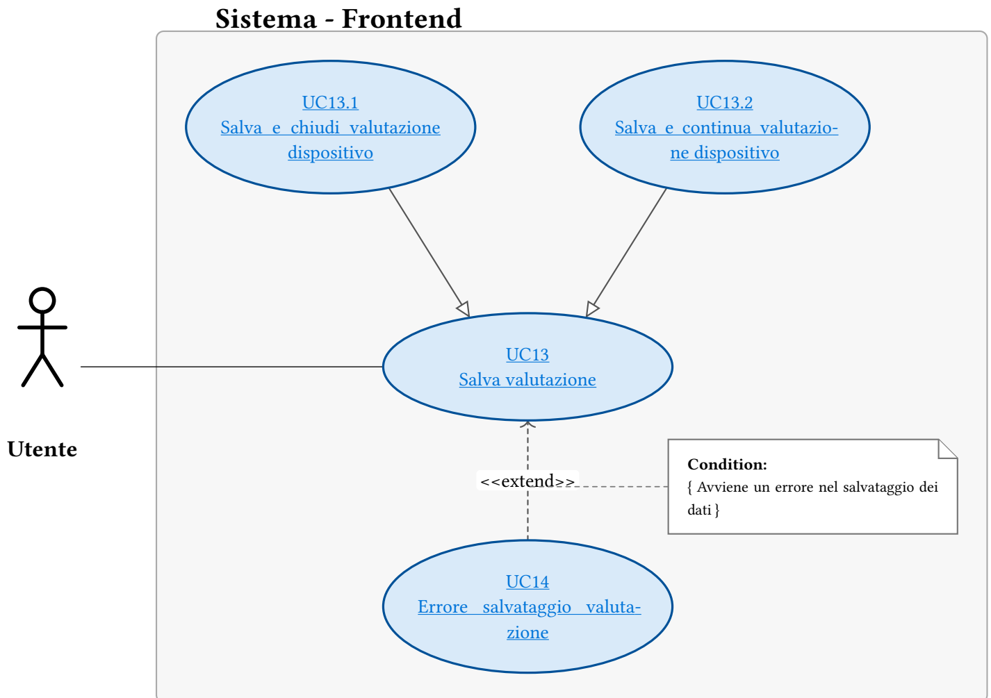
Figura 15: UC13 - Salva valutazione
