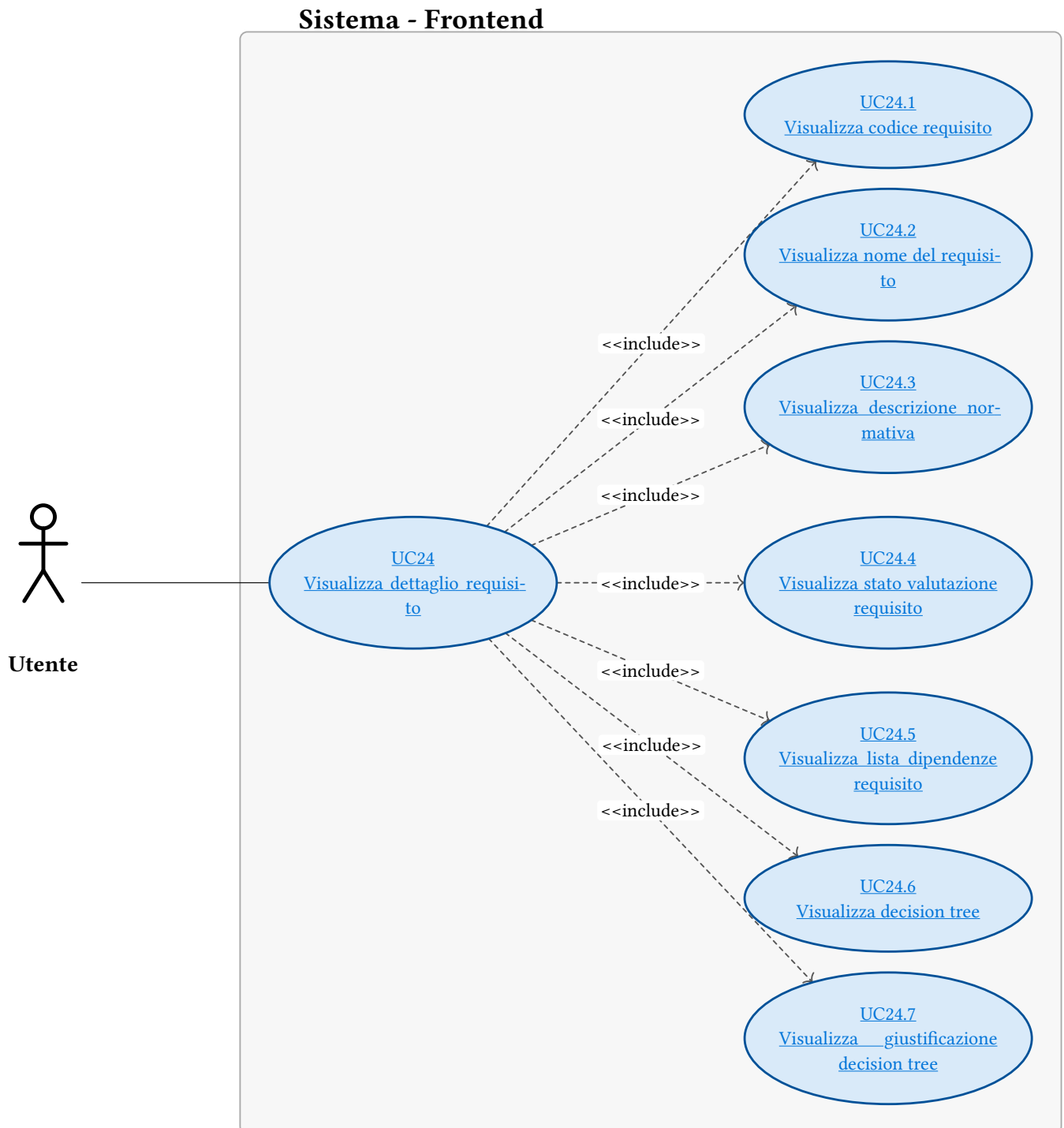
Figura 32: UC24 - Visualizza dettaglio requisito
