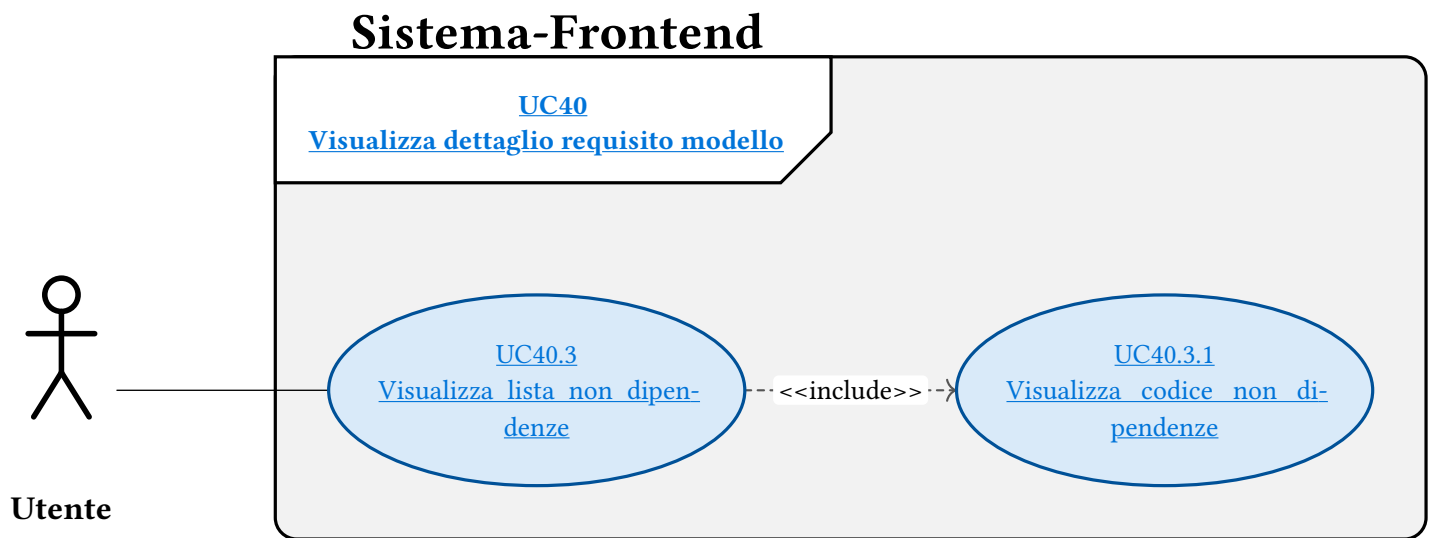
Figura 66: UC40.3 - Visualizza lista non dipendenze
