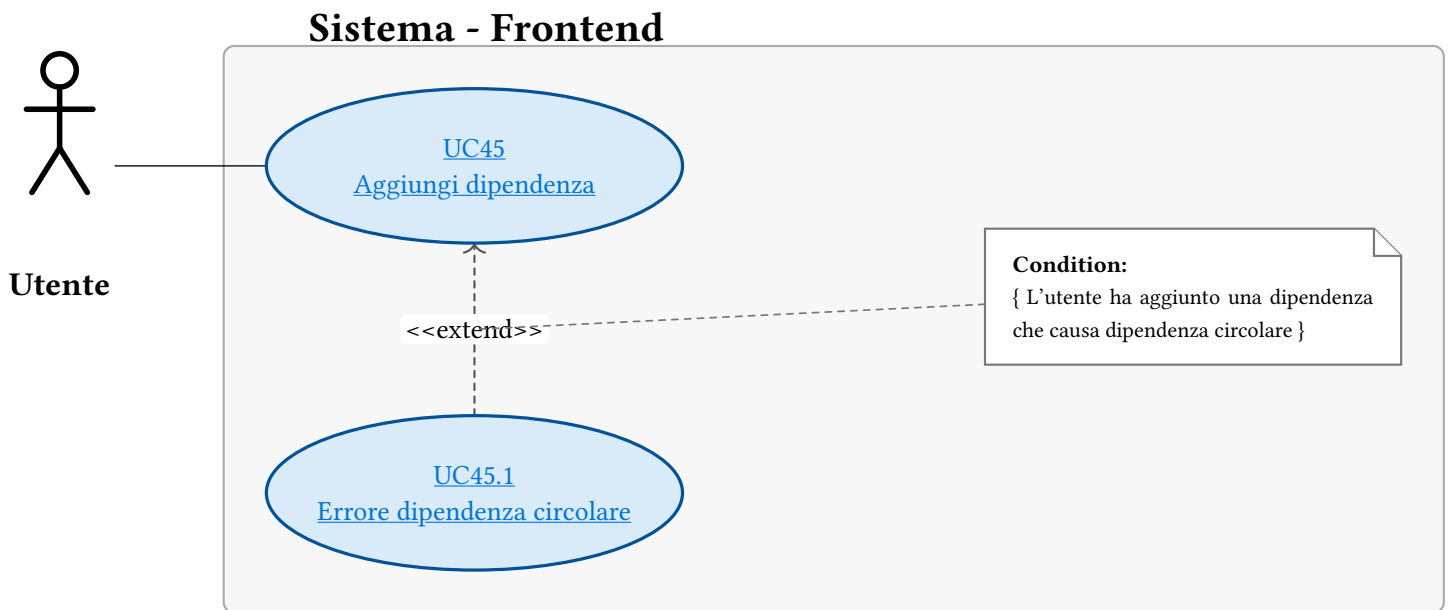
Figura 79: UC45 - Aggiungi dipendenza
