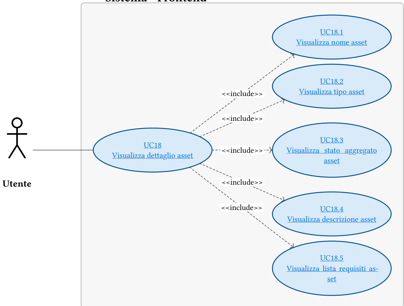
Figura 23: UC18 - Visualizza dettaglio asset
