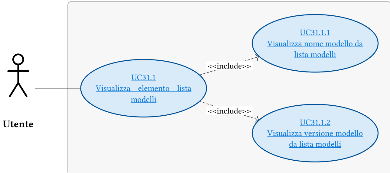
Figura 49: UC31.1 - Visualizza elemento lista modelli
