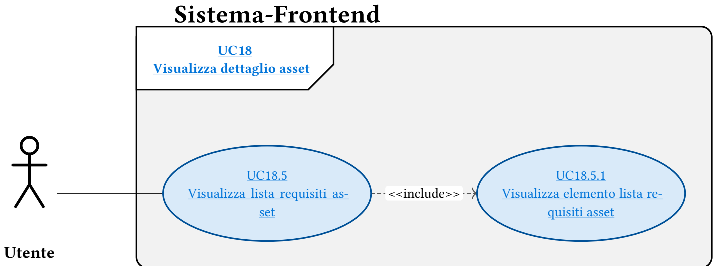
Figura 24: UC18.5 - Visualizza lista requisiti asset
