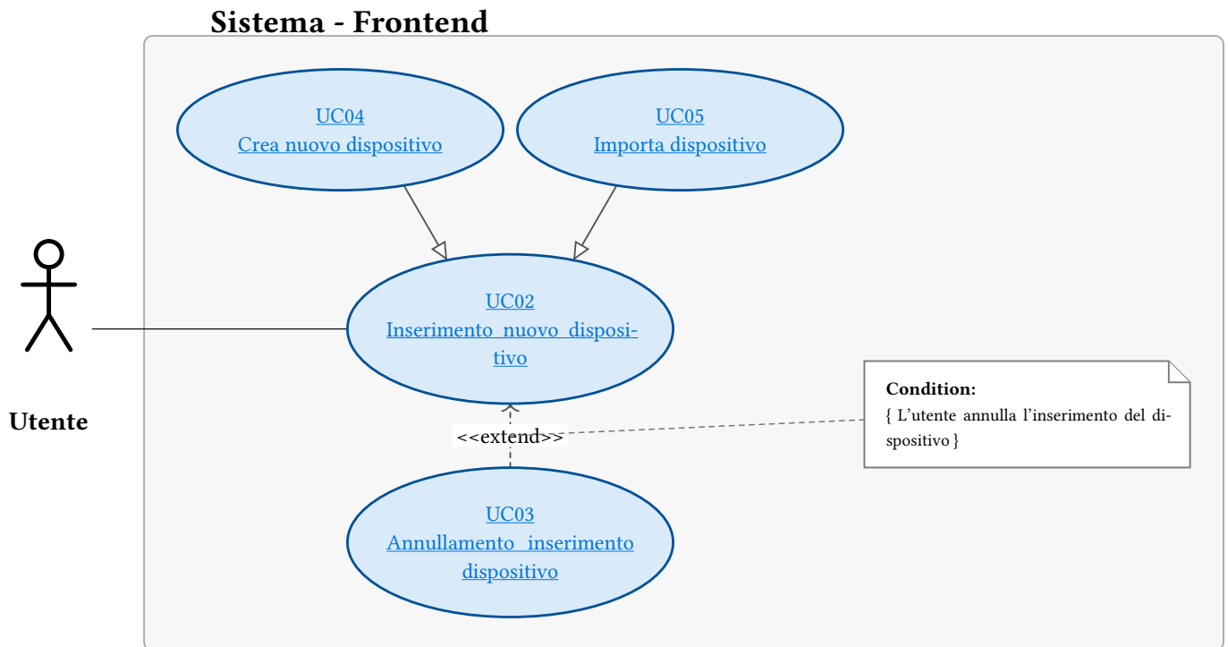
Figura 3: UC02 - Inserimento nuovo dispositivo
