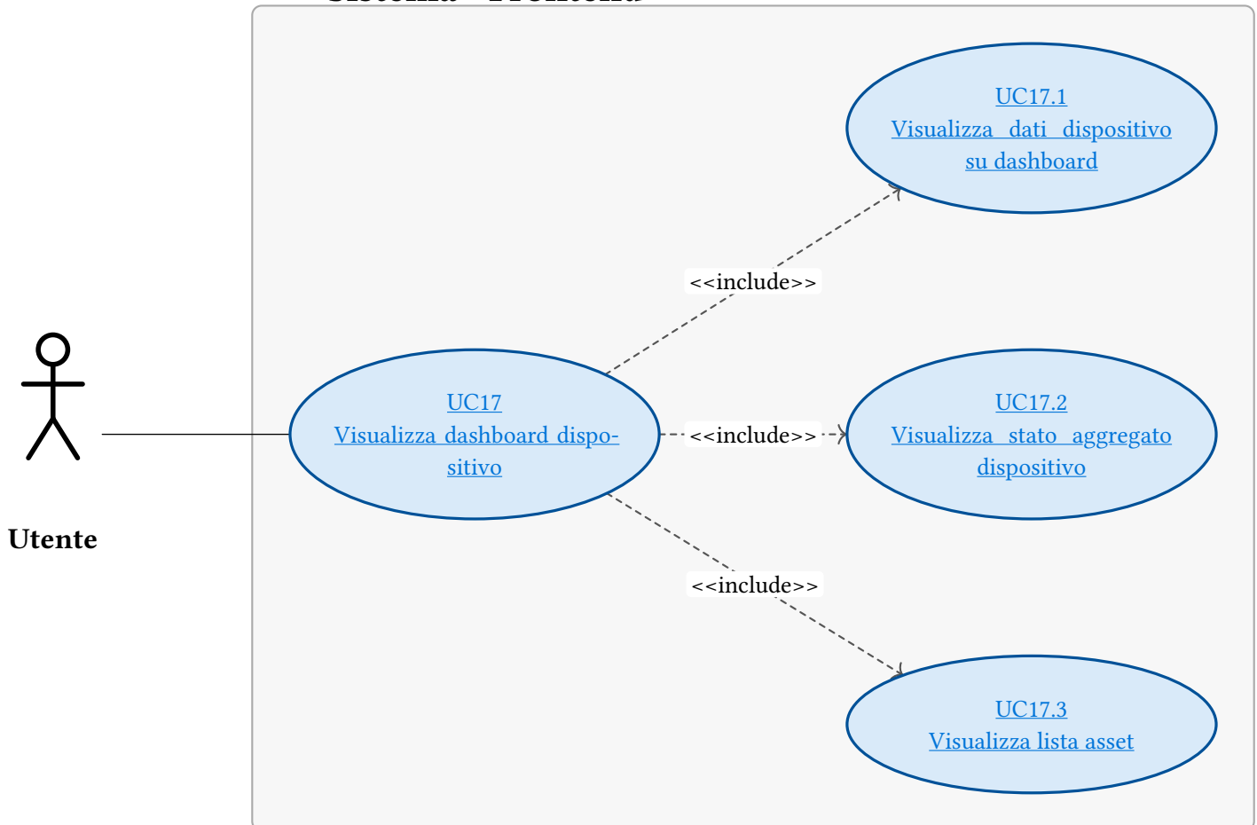
Figura 19: UC17 - Visualizza dashboard dispositivo
