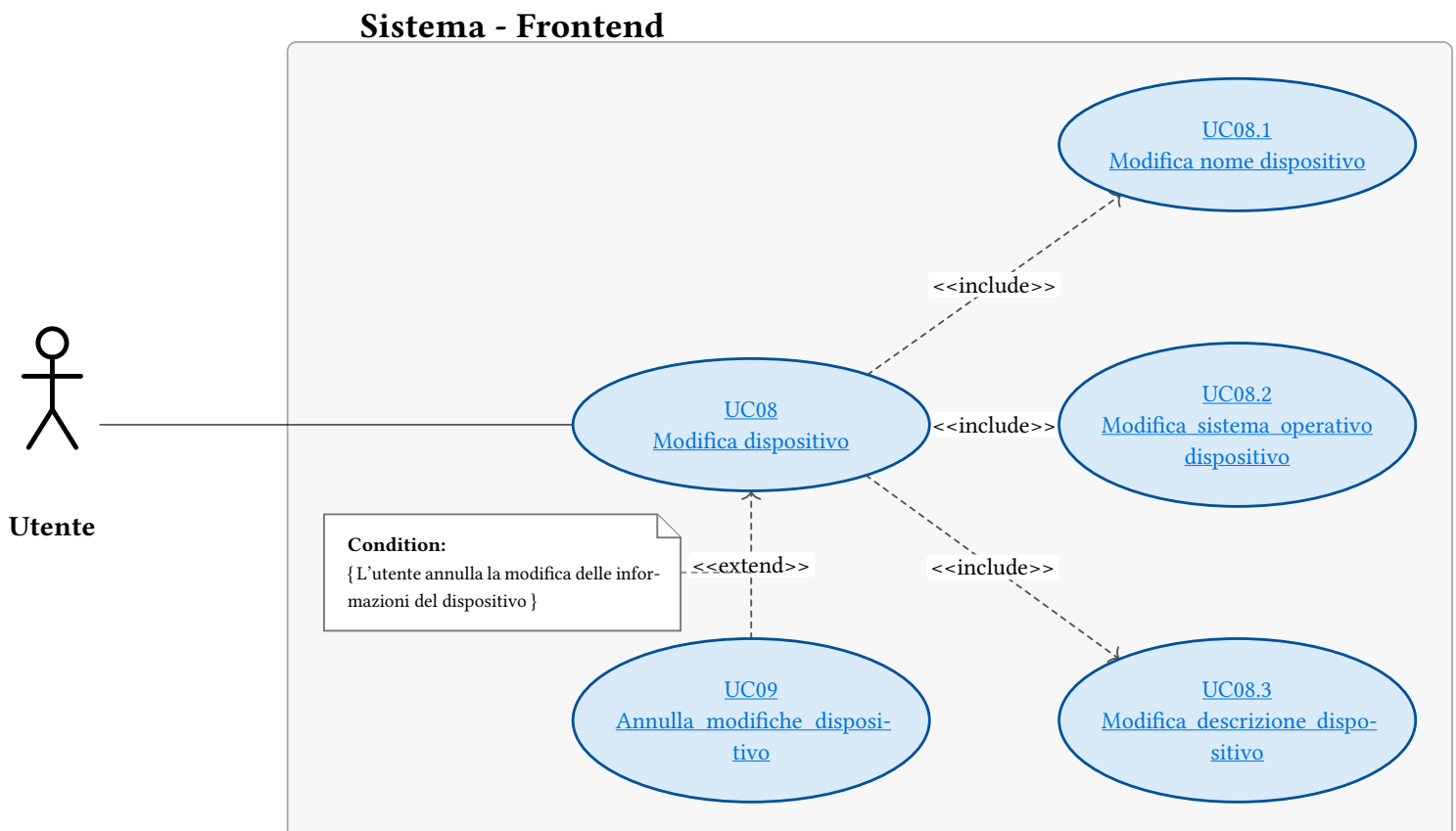
Figura 10: UC08 - Modifica dispositivo
