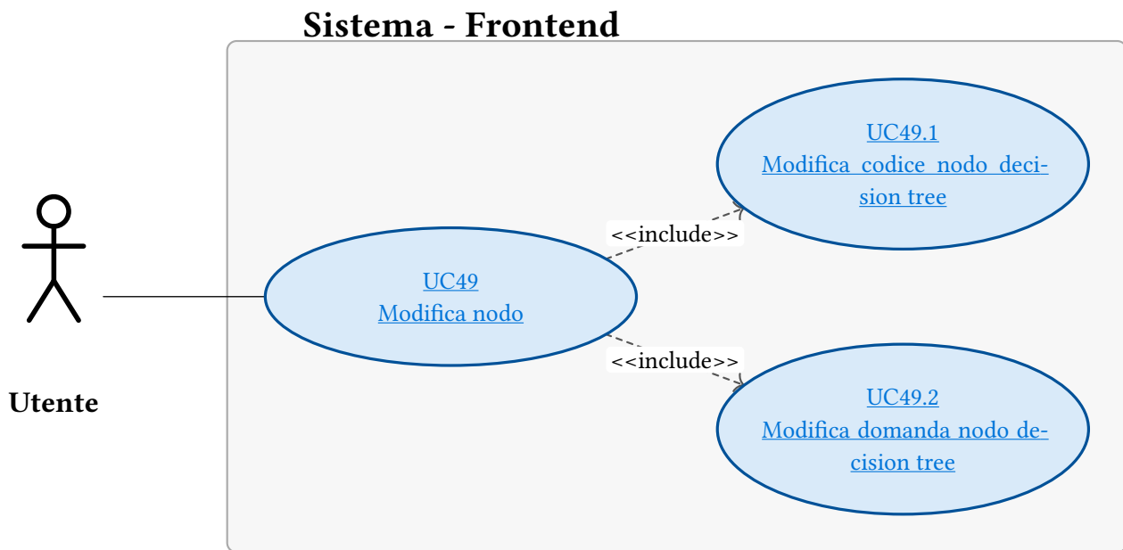
Figura 87: UC49 - Modifica nodo
