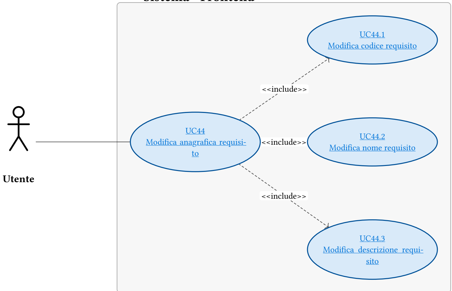
Figura 76: UC44 - Modifica anagrafica requisito
