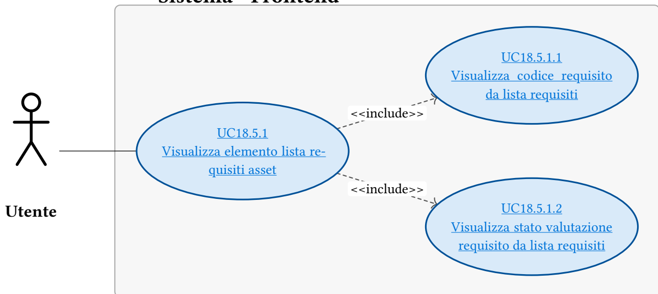
Figura 25: UC18.5.1 - Visualizza elemento lista requisiti asset
