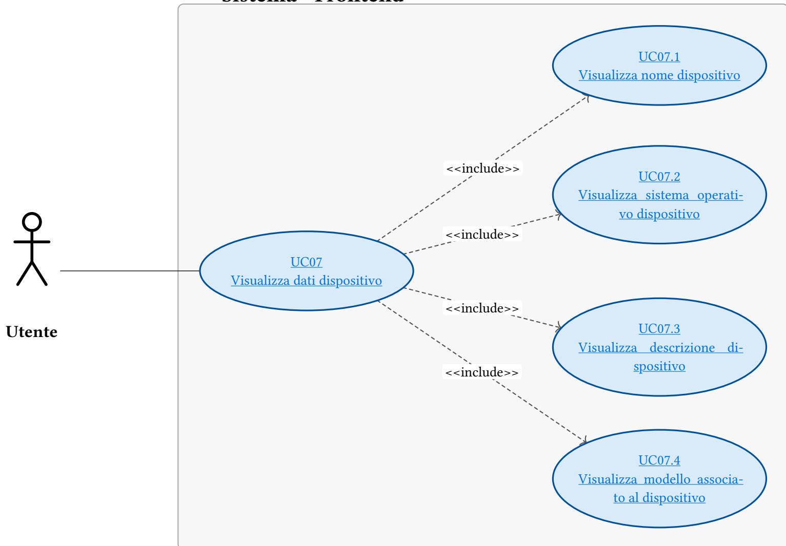
Figura 8: UC07 - Visualizza dati dispositivo
