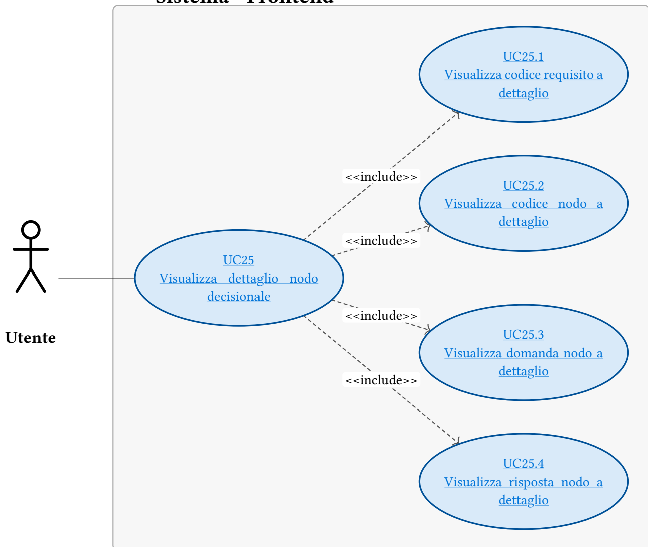
Figura 41: UC25 - Visualizza dettaglio nodo decisionale
