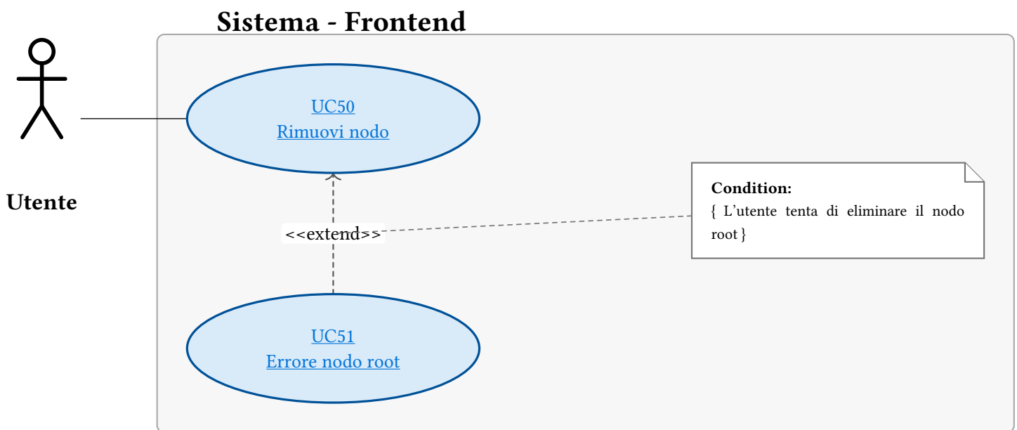
Figura 90: UC50 - Rimuovi nodo
