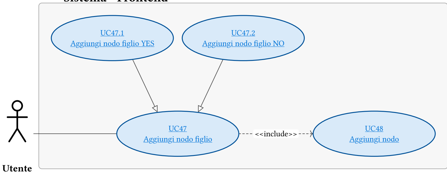
Figura 81: UC47 - Aggiungi nodo figlio
