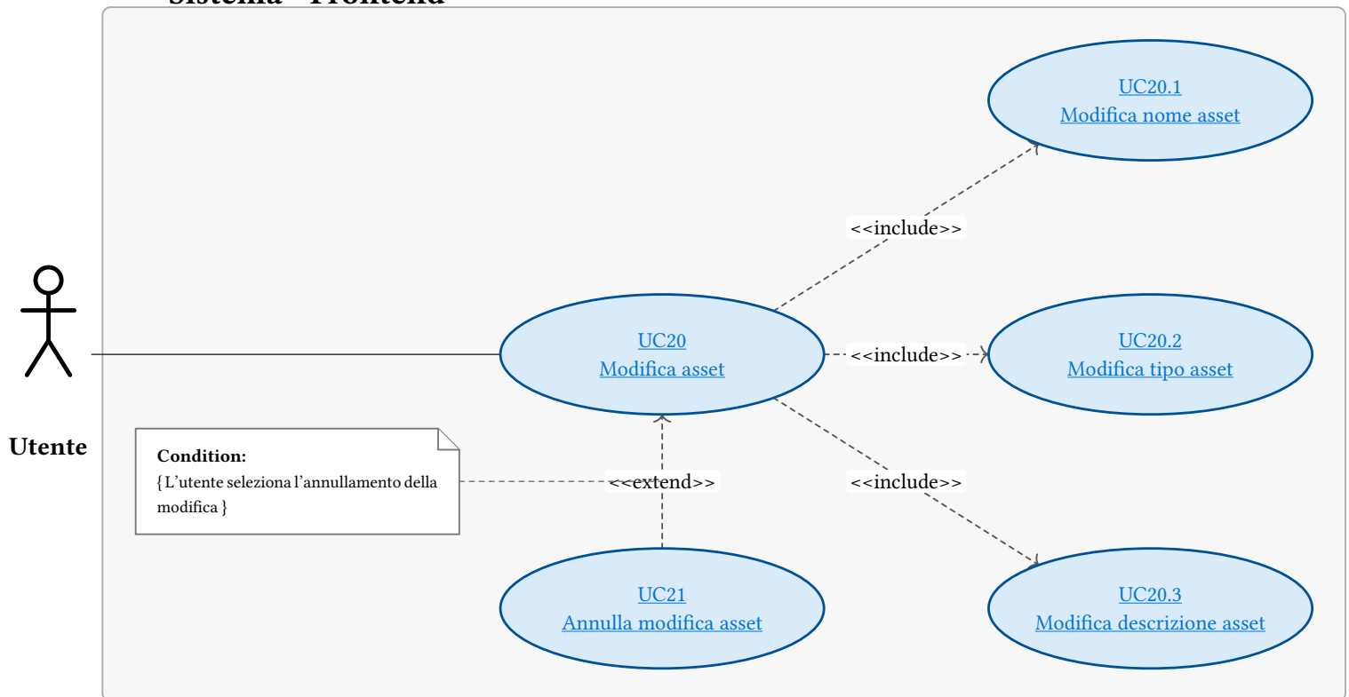
Figura 27: UC20 - Modifica asset
