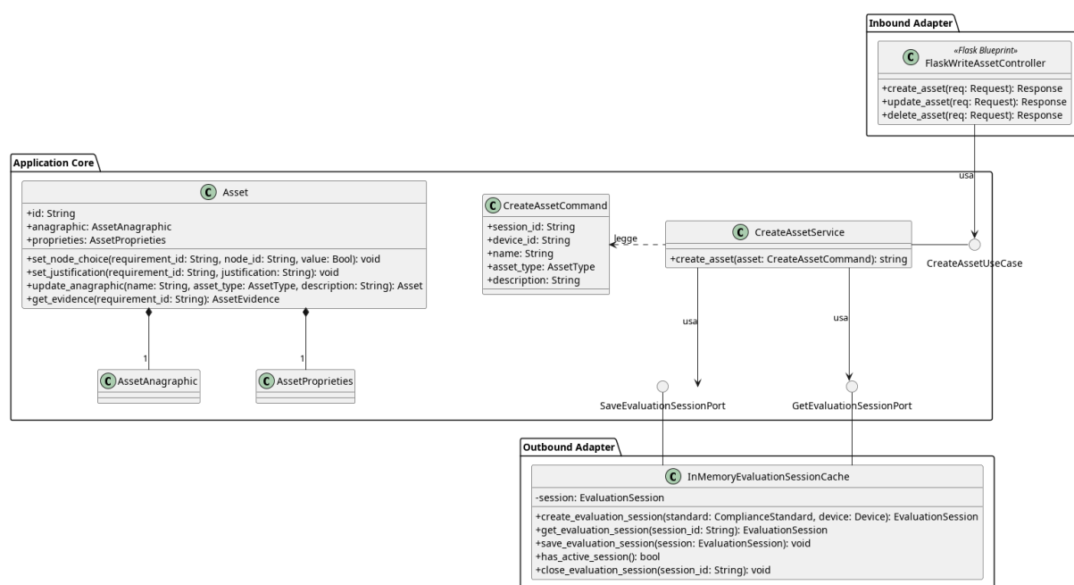
Figura 71: Caso d'uso CreateAsset
