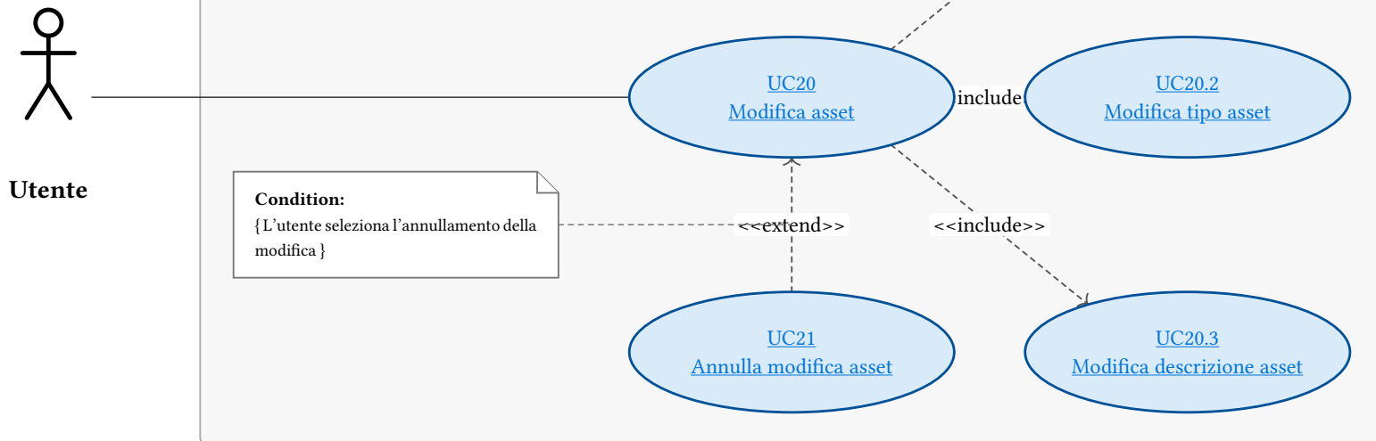
Figura 27: UC20 - Modifica asset
