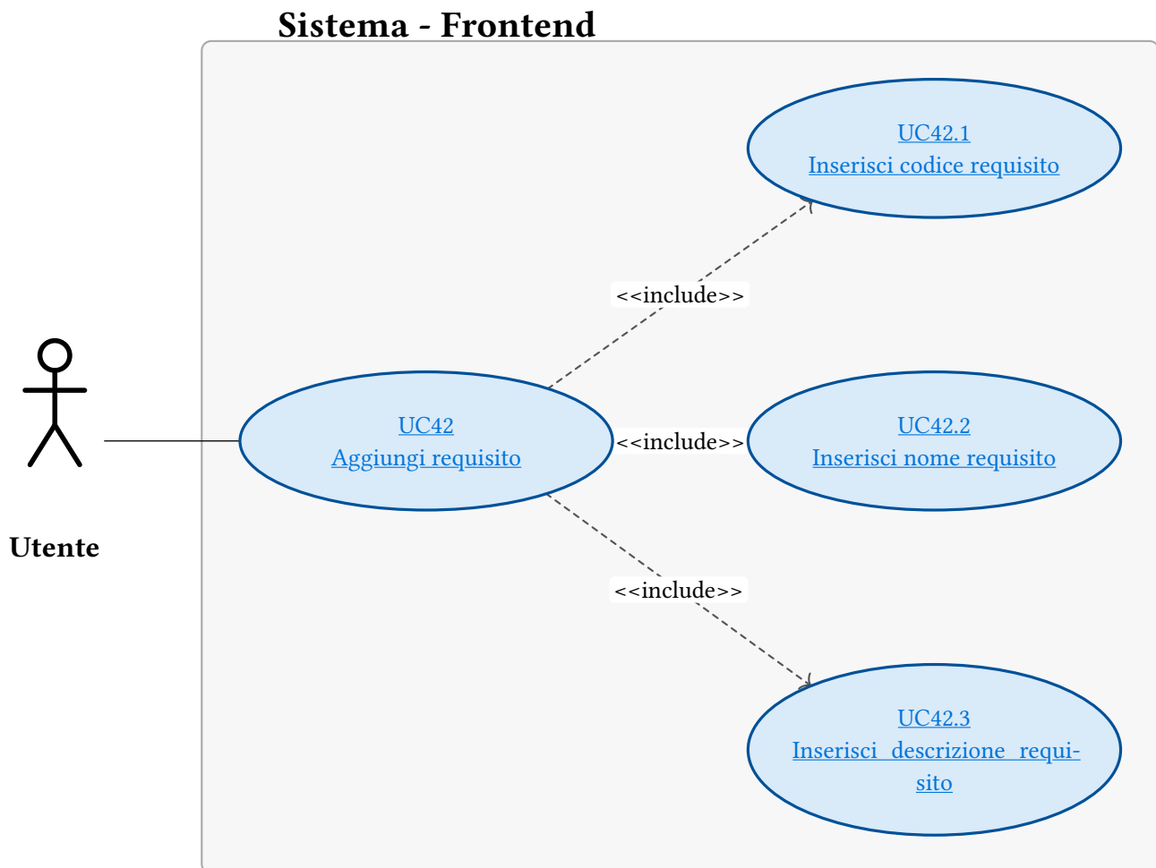
Figura 72: UC42 - Aggiungi requisito
