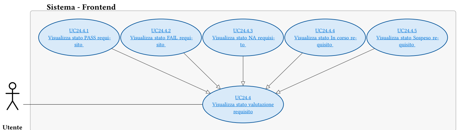
Figura 33: UC24.4 - Visualizza stato valutazione requisito
