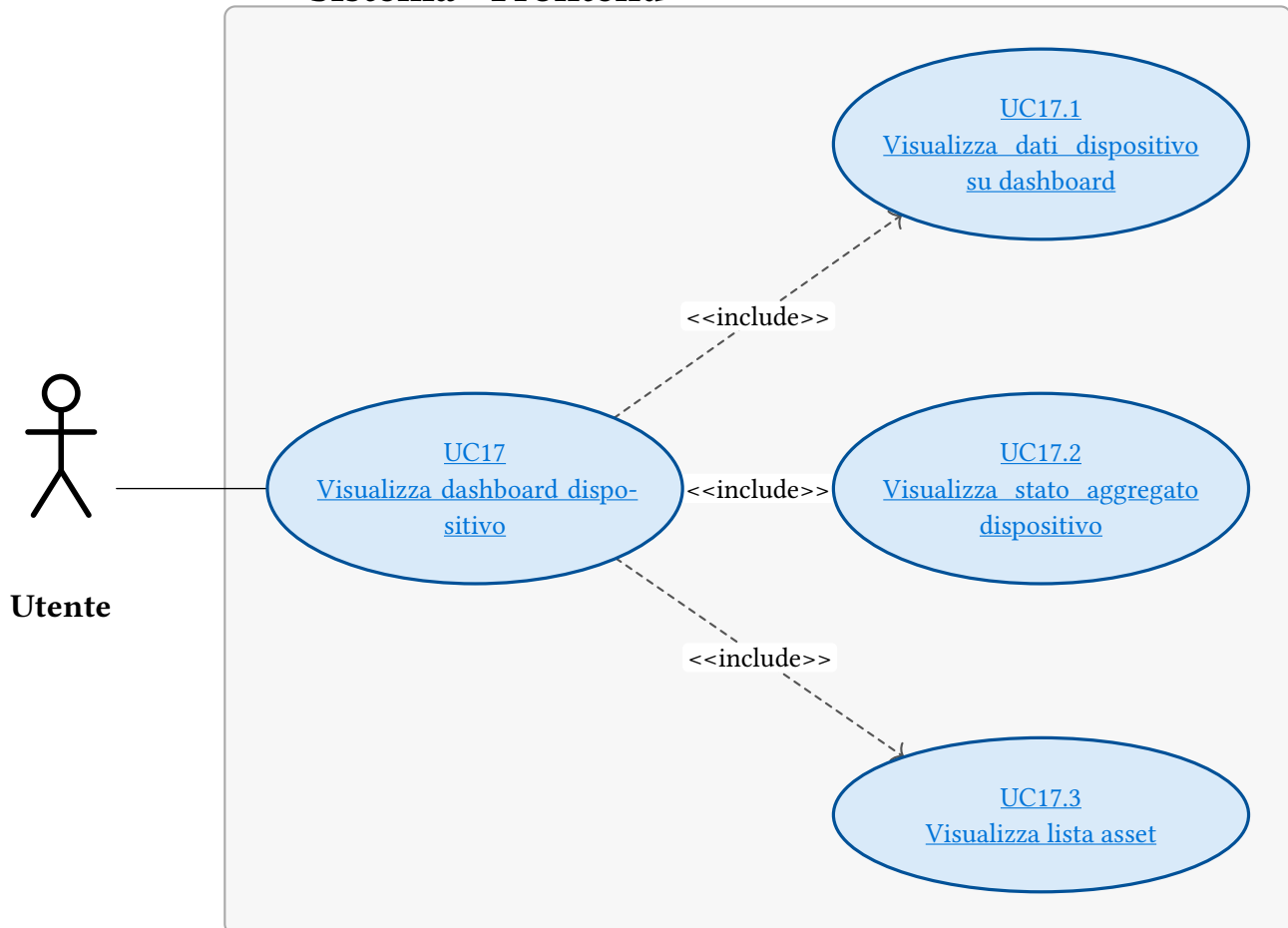
Figura 19: UC17 - Visualizza dashboard dispositivo
