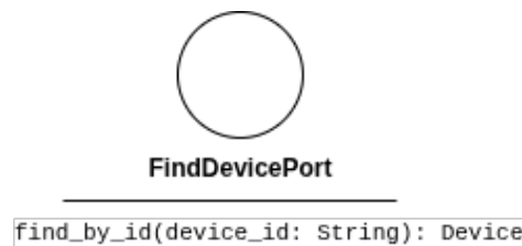
Figura 49: FindDevicePort
