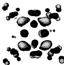
HOMO
