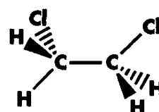
gauche
