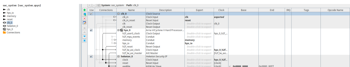
Gambar 6. Platform Designer: HPS, lightweight AXI, dan HEKETON dalam sistem Qsys.
