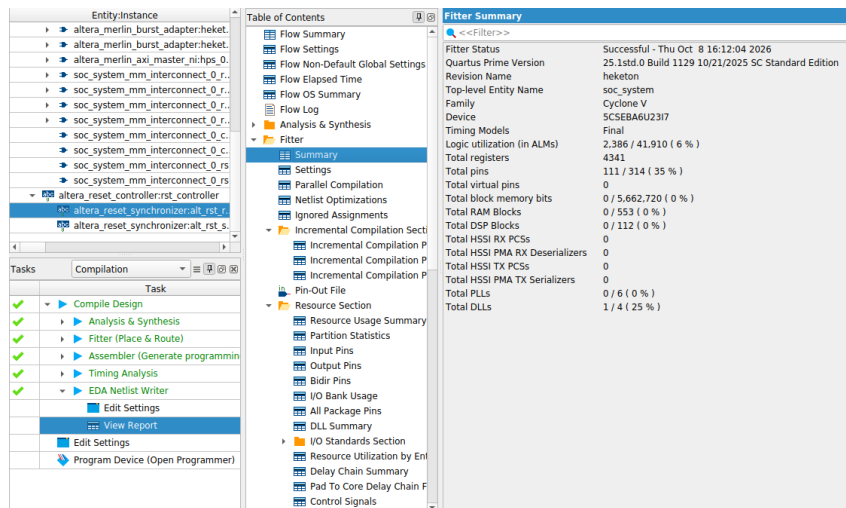
Gambar 4. Fitter Summary: status kompilasi berhasil dan ringkasan penggunaan sumber daya pada Cyclone V.
